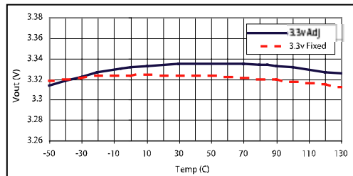
图 12 VIN=5.0V, IOUT=10mA
