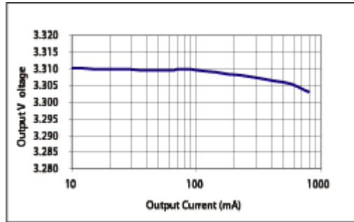
图 1 SPX1117M3-3.3 负载调节率; V_{IN}=4.8V
