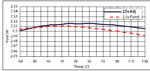
图 9 VIN=4.0V, IOUT=10mA
