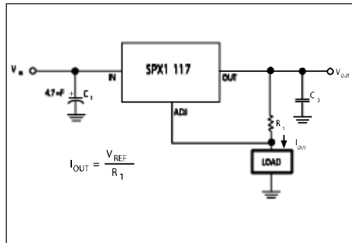
图 21 电流源
