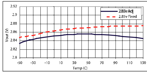
图 10 VIN=4.85, IOUT=10mA
