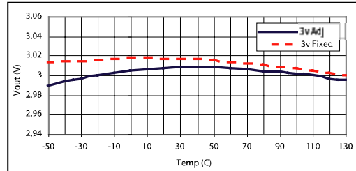
图 11 VIN=4.85, IOUT=10mA
