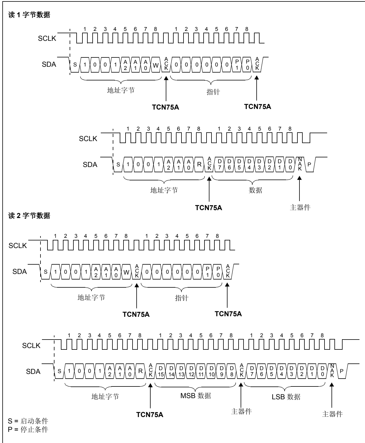
图 5-2: 从寄存器中读取 1 个字节和 2 个字节的数
