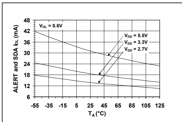
图 2-7: ALERT 和 SDA 的 I_{OL} ——环境温度曲线
