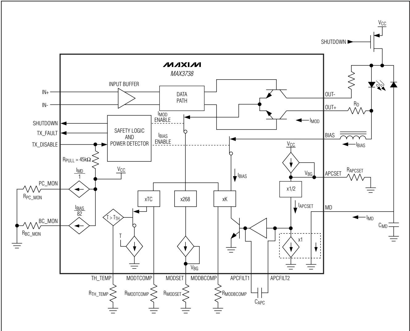
图4. 功能图
