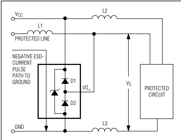
图6. 布局考虑
