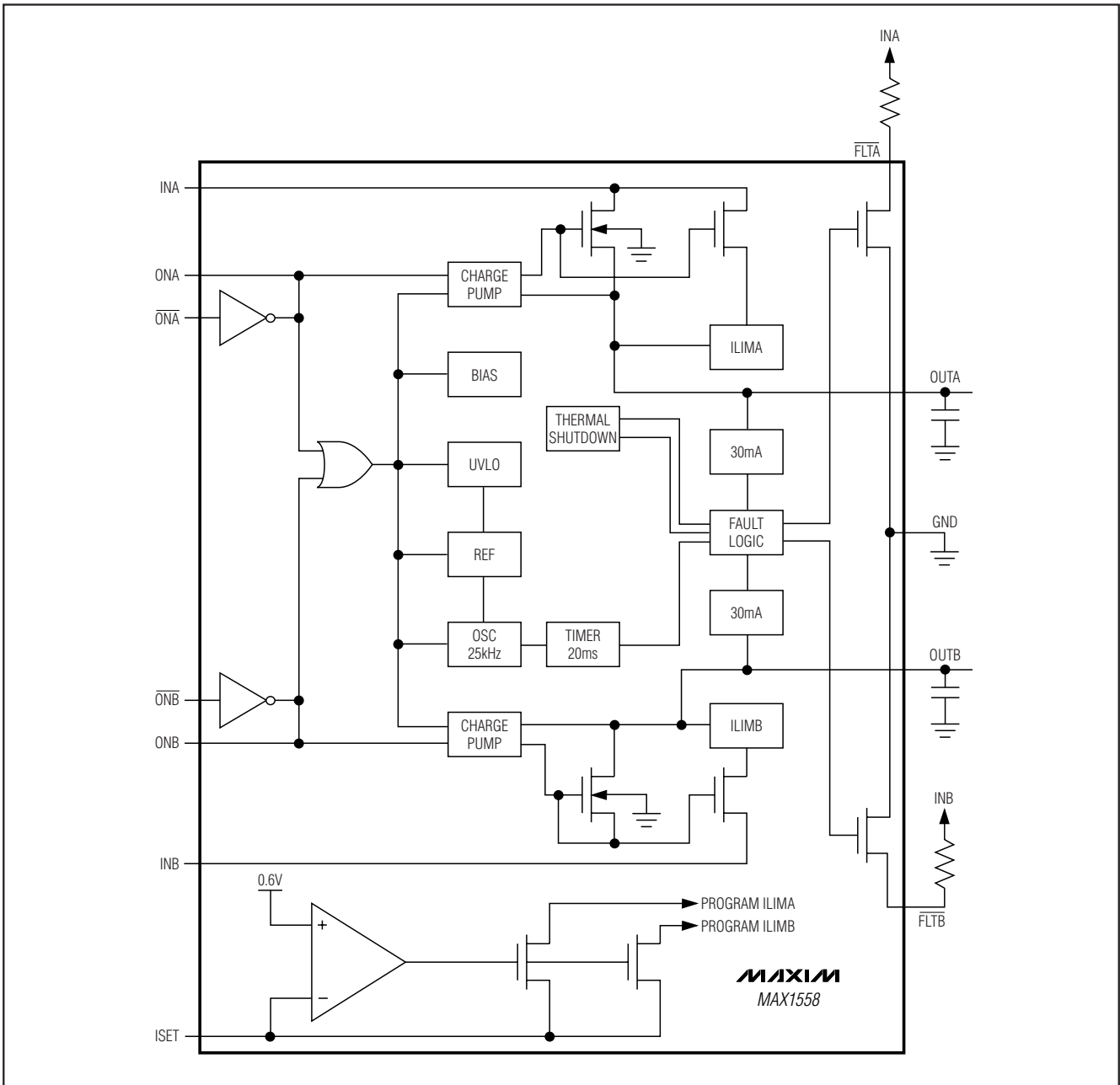
图 2. 功能框图
