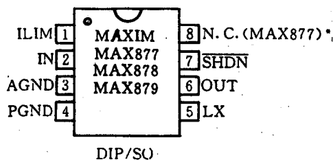
图 2 MAX877/878/879 引脚排列 *
