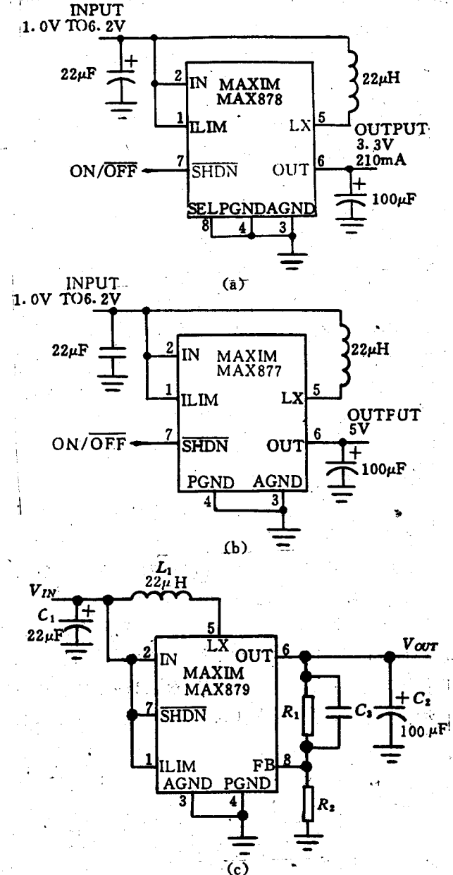
图 4 MAX877/878/879/典型应用电路
