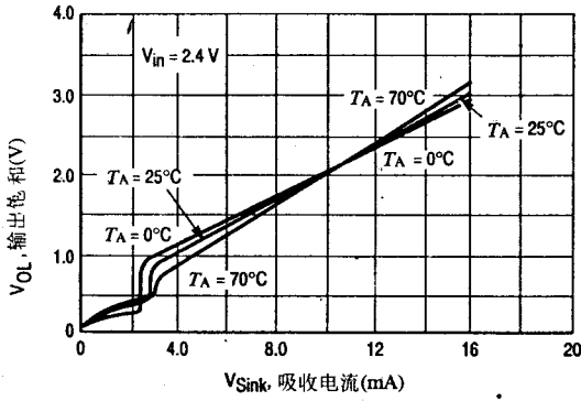
图 4.366 MC3X164-3 复位输出饱和与吸收电流的关系
