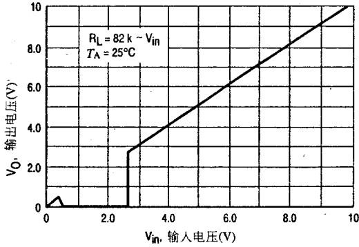
图 4.358 MC3X164-3 低有效复位输出电压与输入电压的关系
