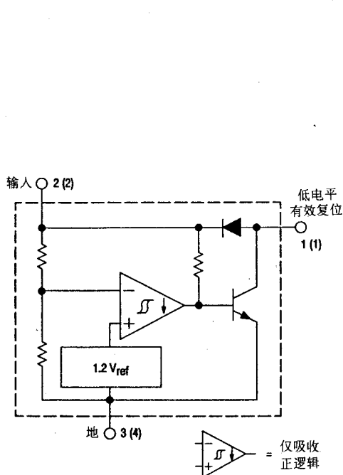
图 4.356 原理图
