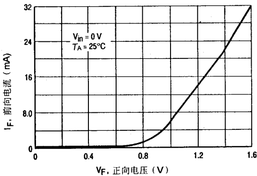
图 4.368 箝位二极管正向电流与电压的关系
