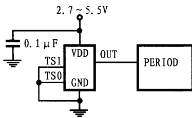
图2 MAX6577与单片机的连接
