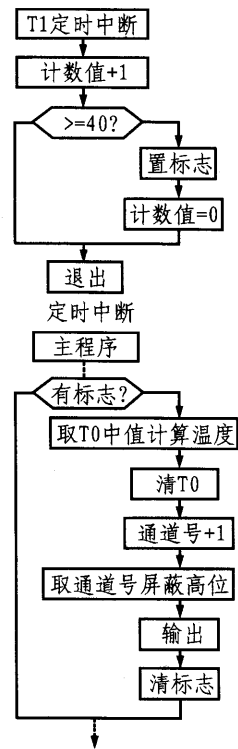
图4 程序流程
