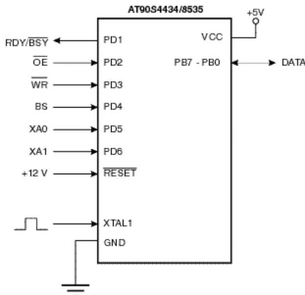
图 67 并行编程
