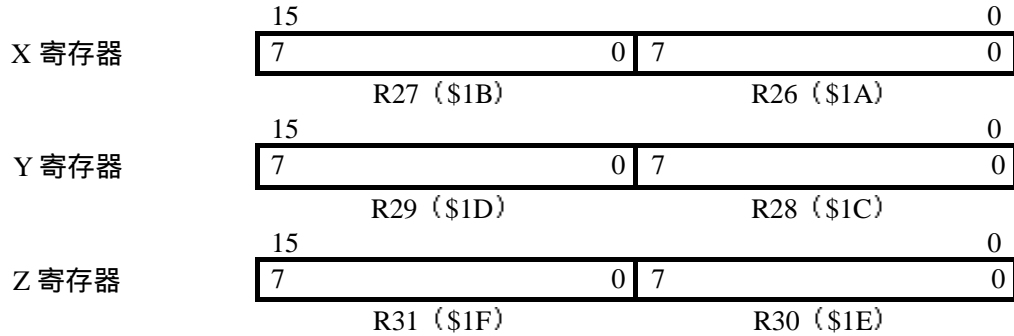
图 7 X、Y、Z 寄存器
