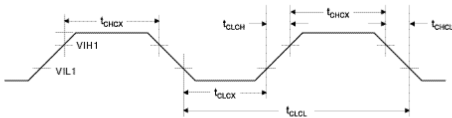
图 74 外部时钟
