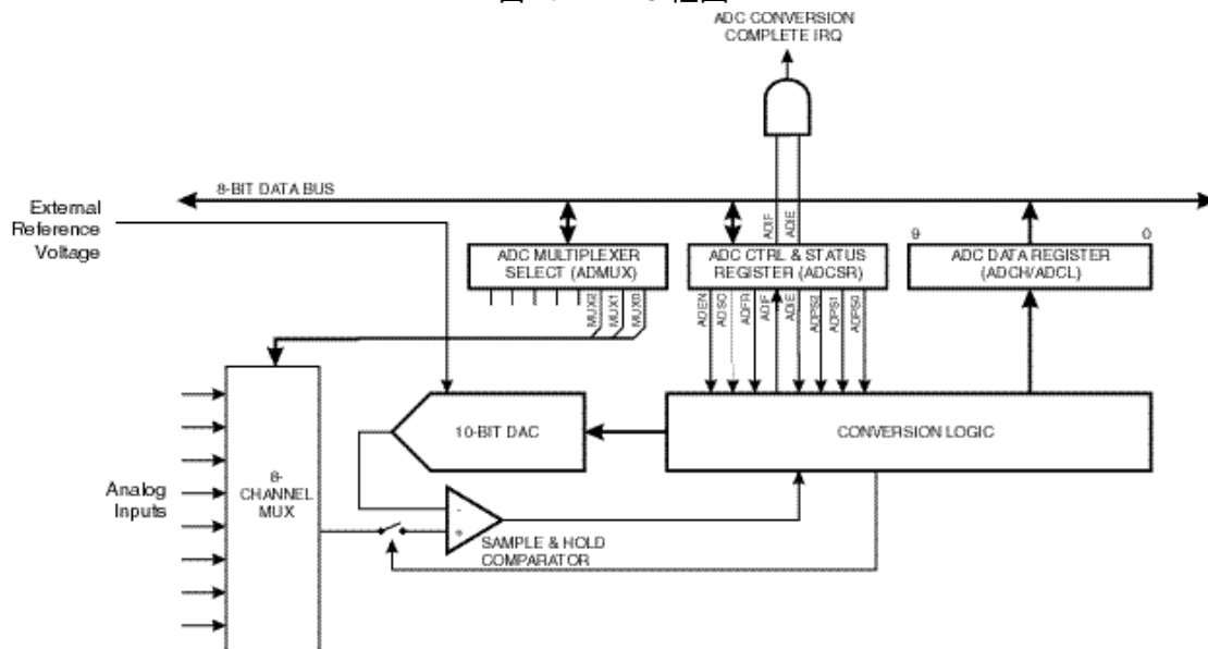
图 45 ADC 框图
