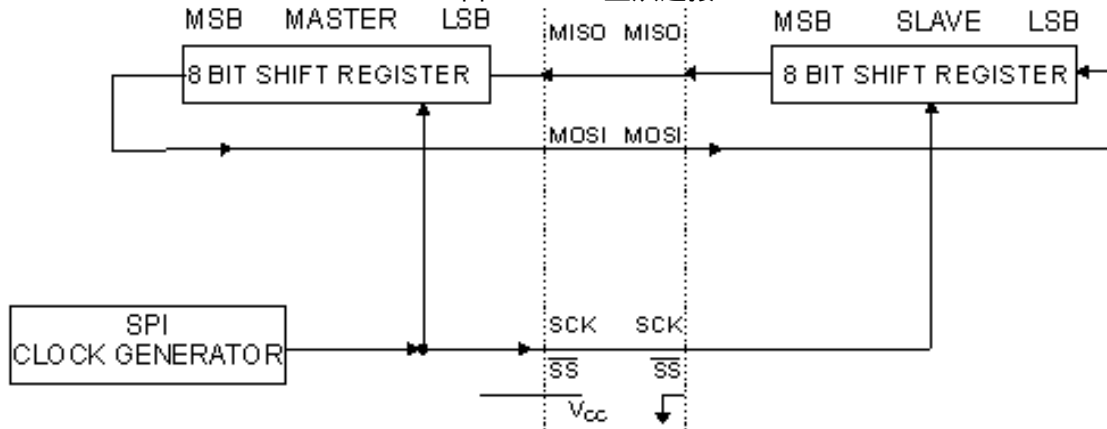
图 38 SPI 主从连接
