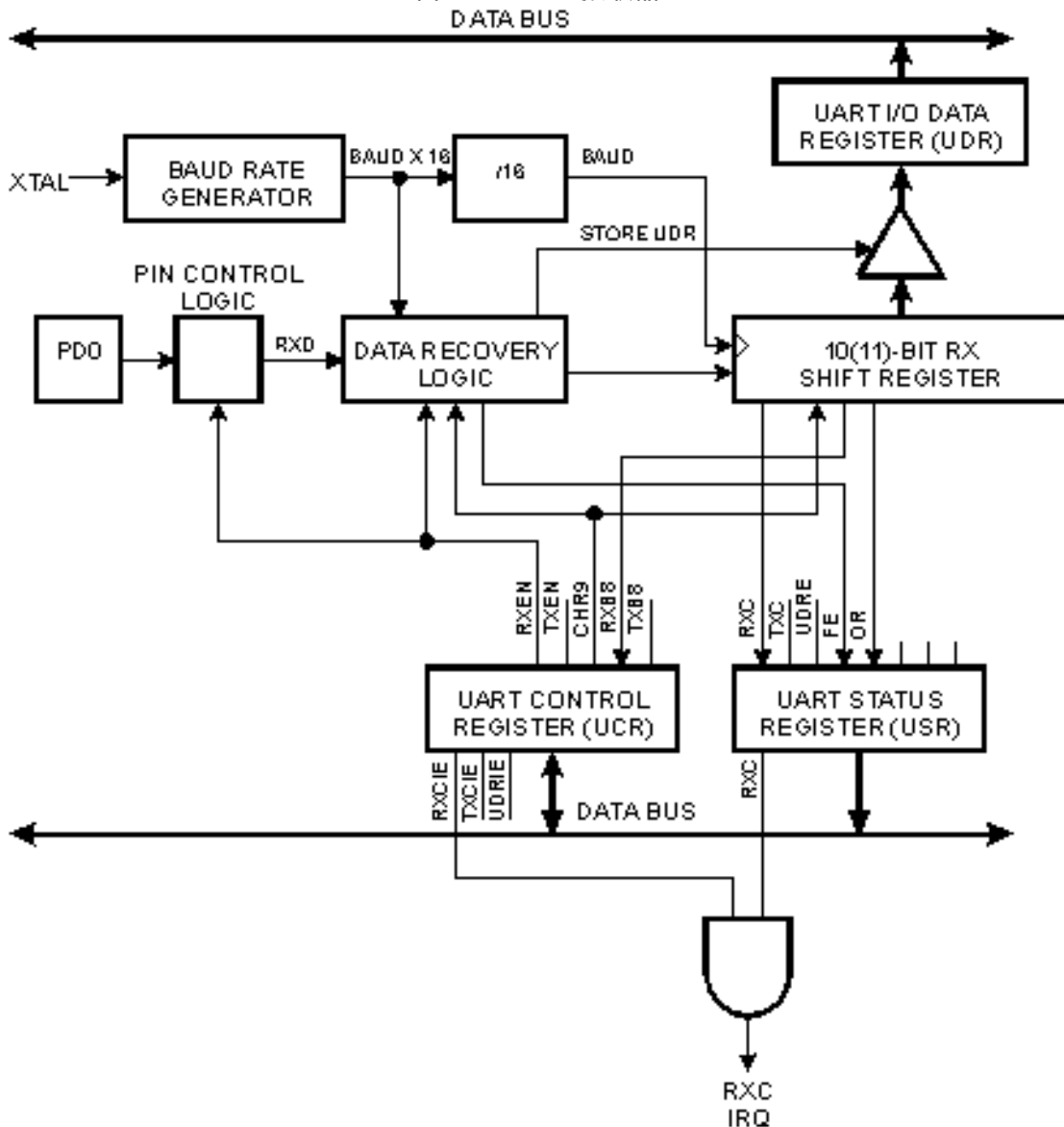
图 42 UART 接收器
