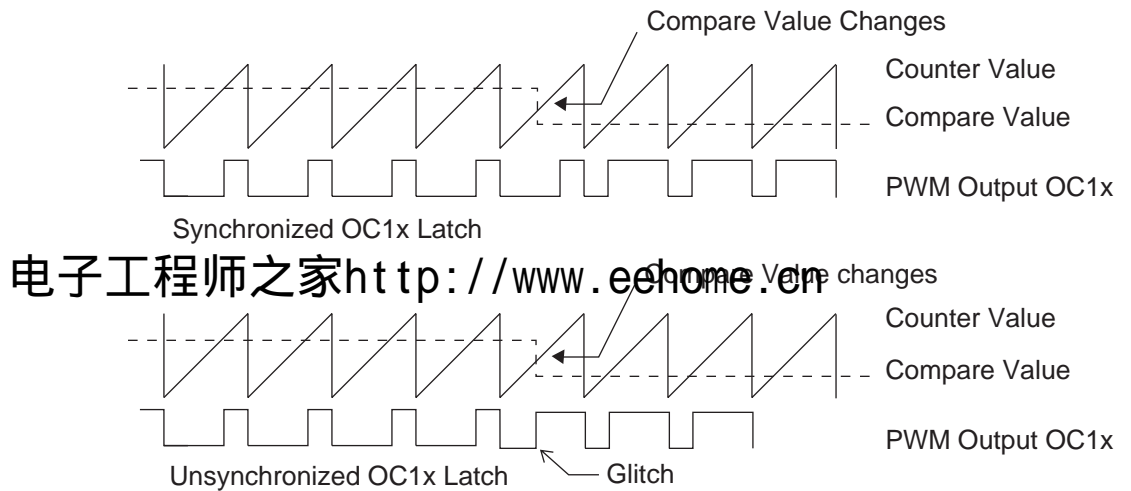
Figure 37. 非同步 OCR 锁存结果
