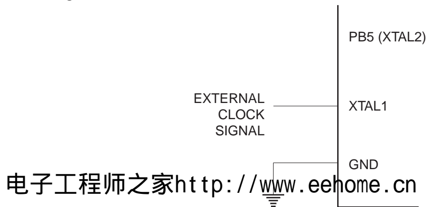
Figure 30. 外部时钟配置图
