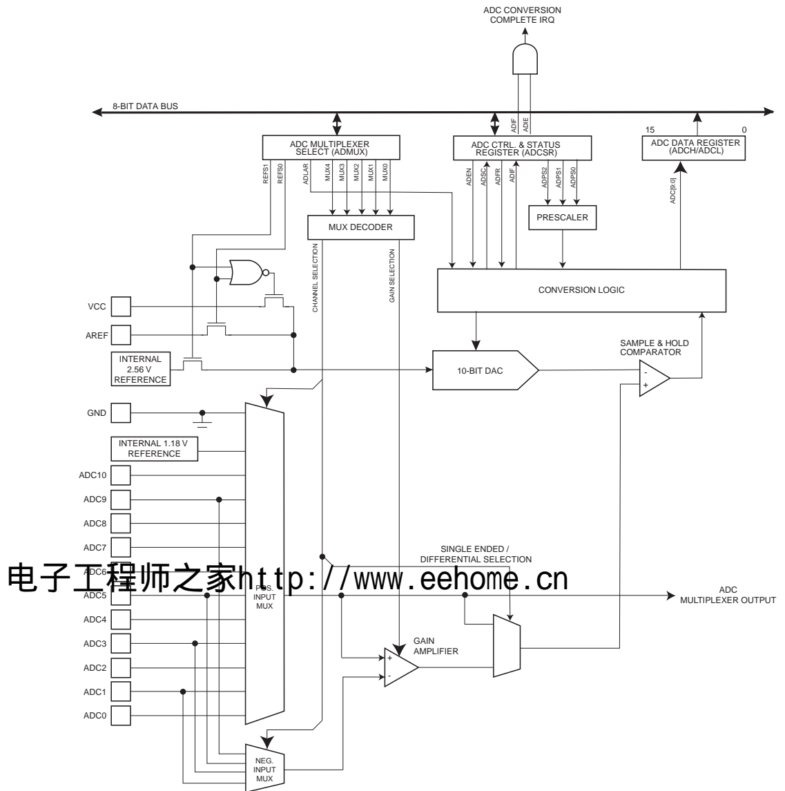
Figure 46. 模数转换器方框图
