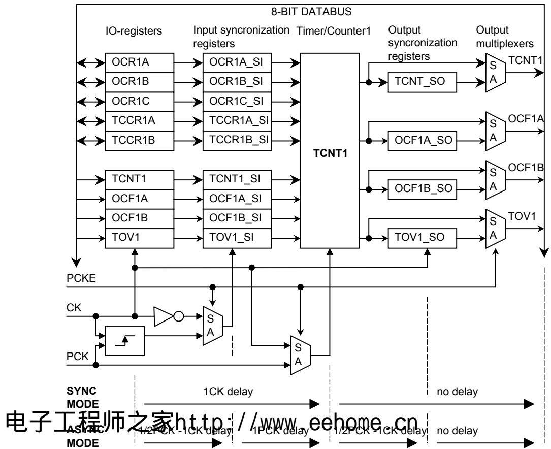
Figure 34. T/C1 同步寄存器方框图
