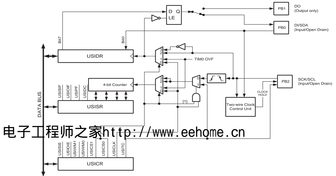
Figure 39. 通用串行接口框图
