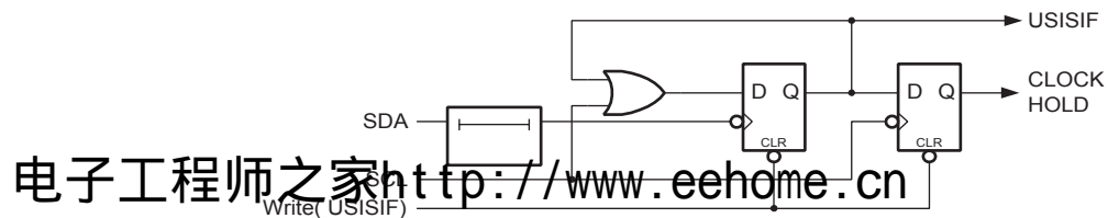
Figure 44. 起始条件监测器逻辑电路图
