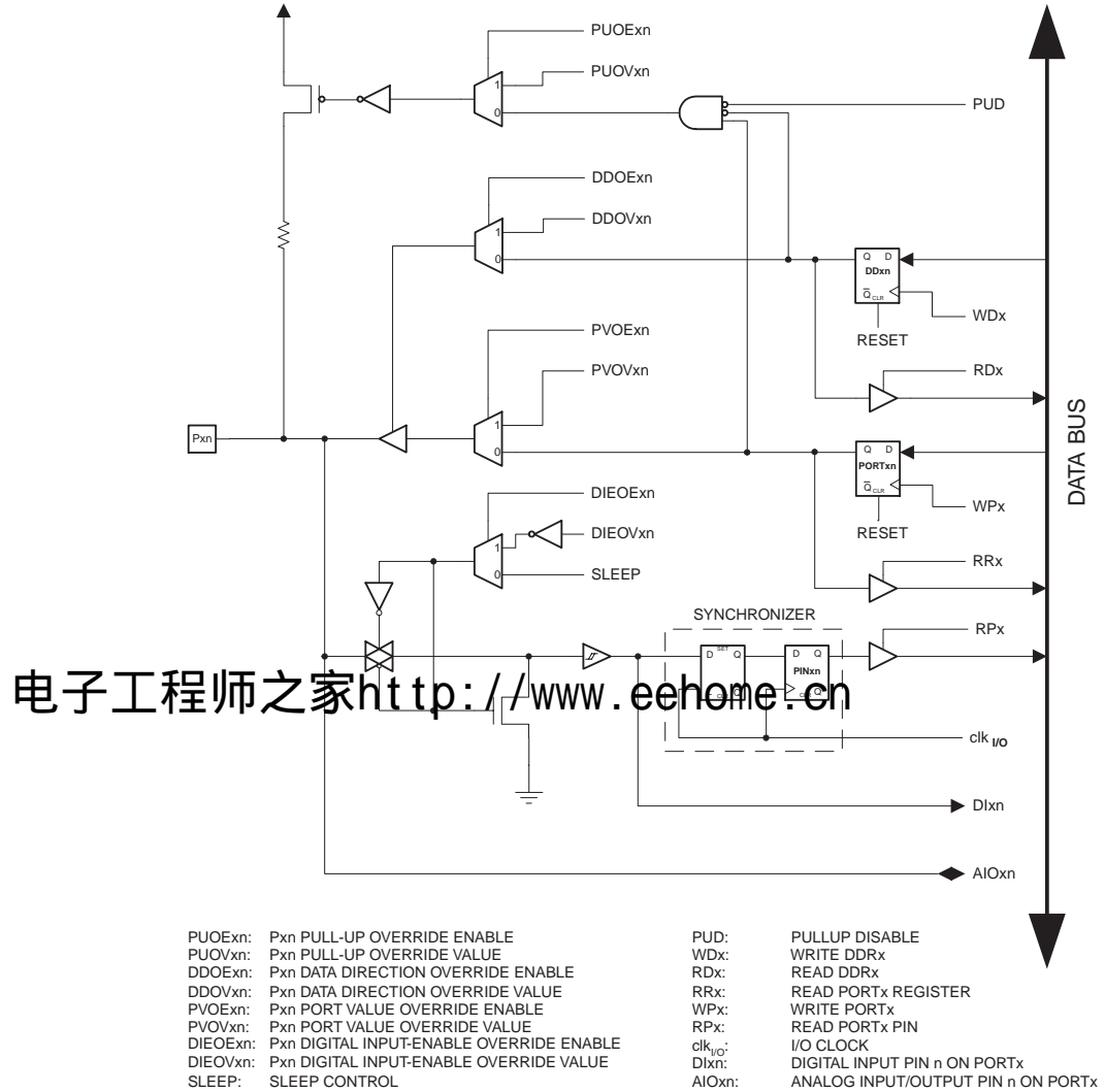
Figure 57. 端口的第二功能 (1)
