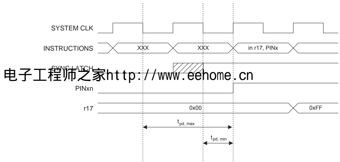
Figure 55. 读取引脚数据时的同步
