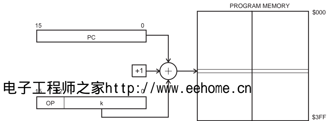
Figure 16. 相关程序存储器寻址
