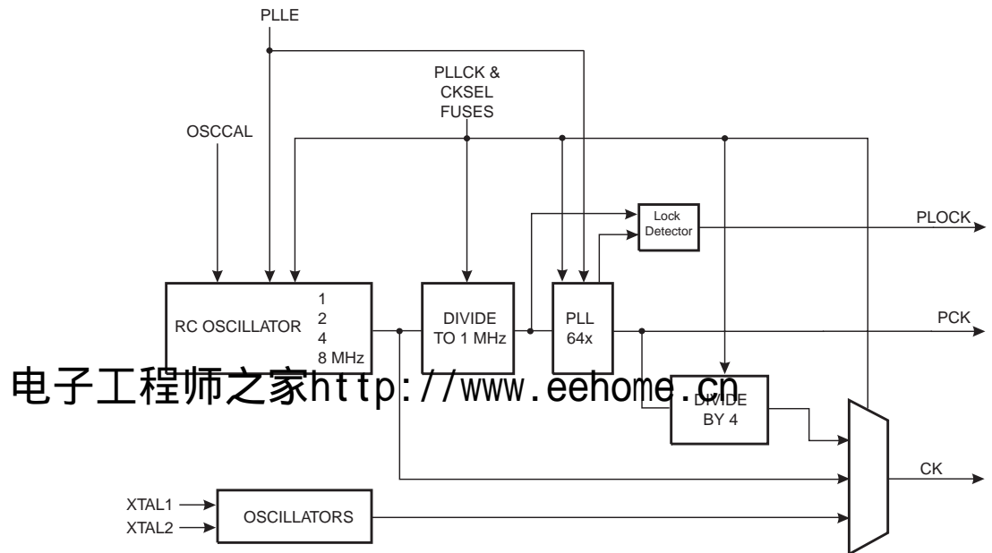
Figure 27. PCK 时钟系统
