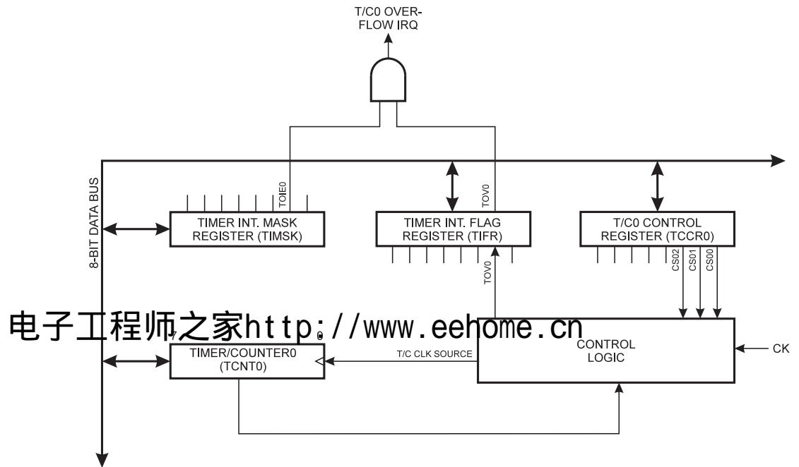
Figure 33. T/C0 方框图
