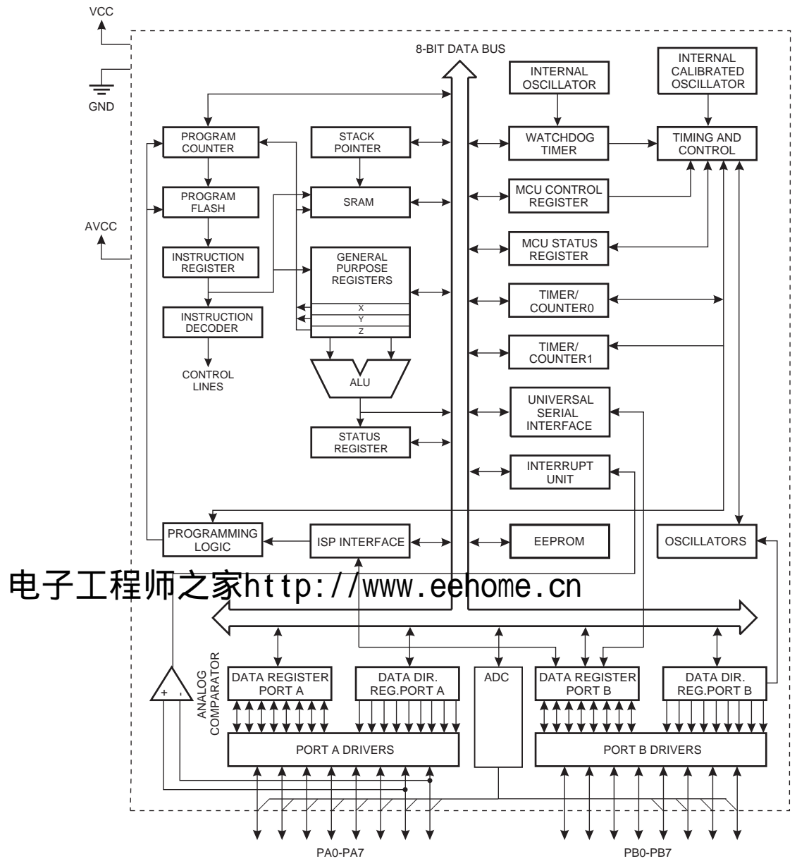
Figure 1. ATtiny26(L) 结构框图
