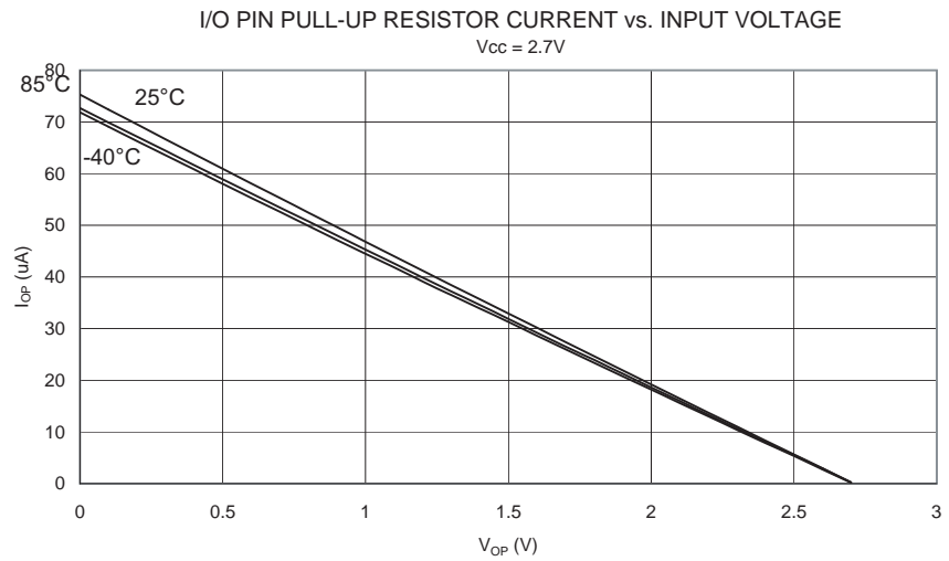
Figure 99. 复位 (Reset) 引脚上拉电阻电流和 Reset 引脚电压的关系 ( V_{CC} = 5V )
