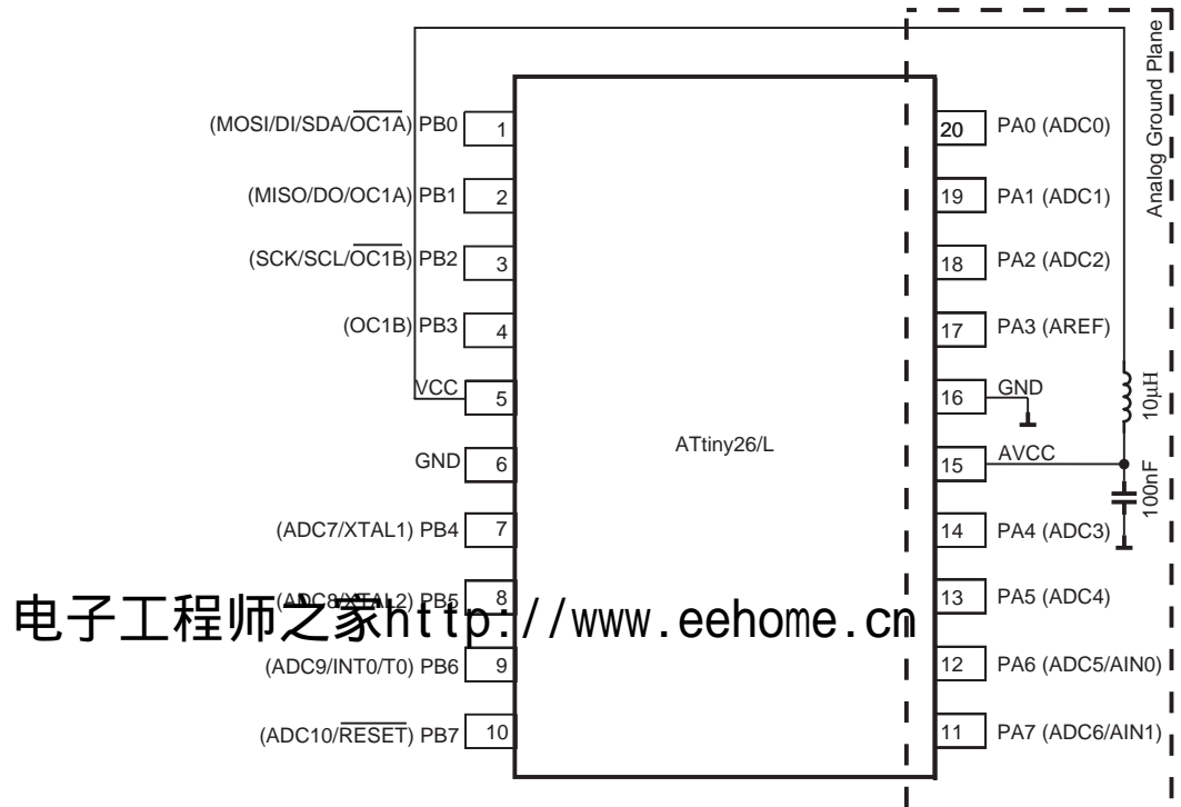
Figure 52. ADC 电源连接图
