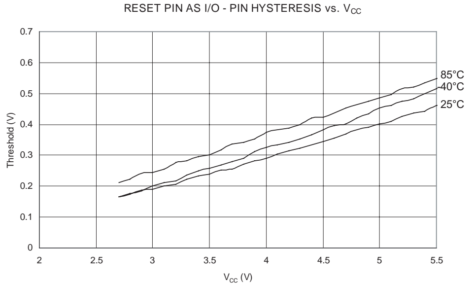
Figure 114. Reset 输入迟滞和 V_{CC} 的关系
