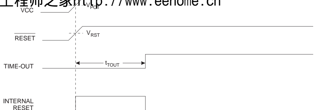
Figure 22. 外部控制 MCU 启动 \overline{\text{RESET}}
