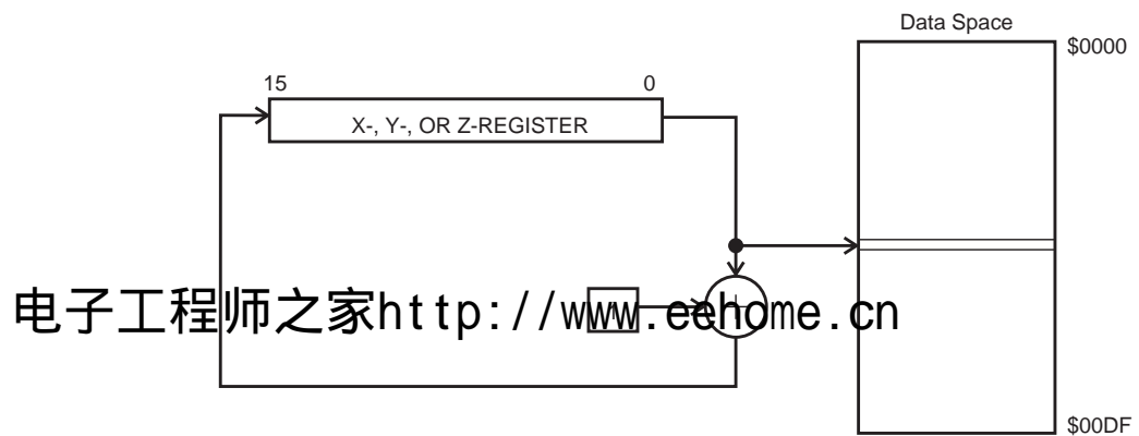
Figure 13. 带后增量的间接数据寻址
