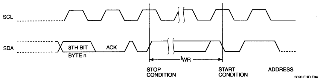
图 2 写周期时序
