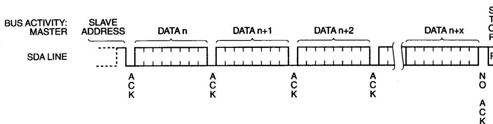
图 10 连续读时序
