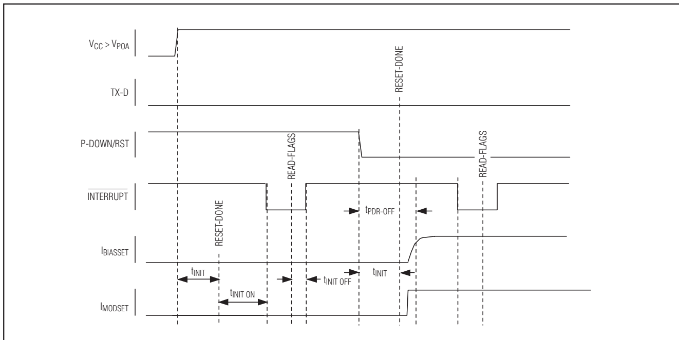
图1. 触发P-DOWN/RST、TX-D/SOFT-TX-D没有触发时的上电初始化
