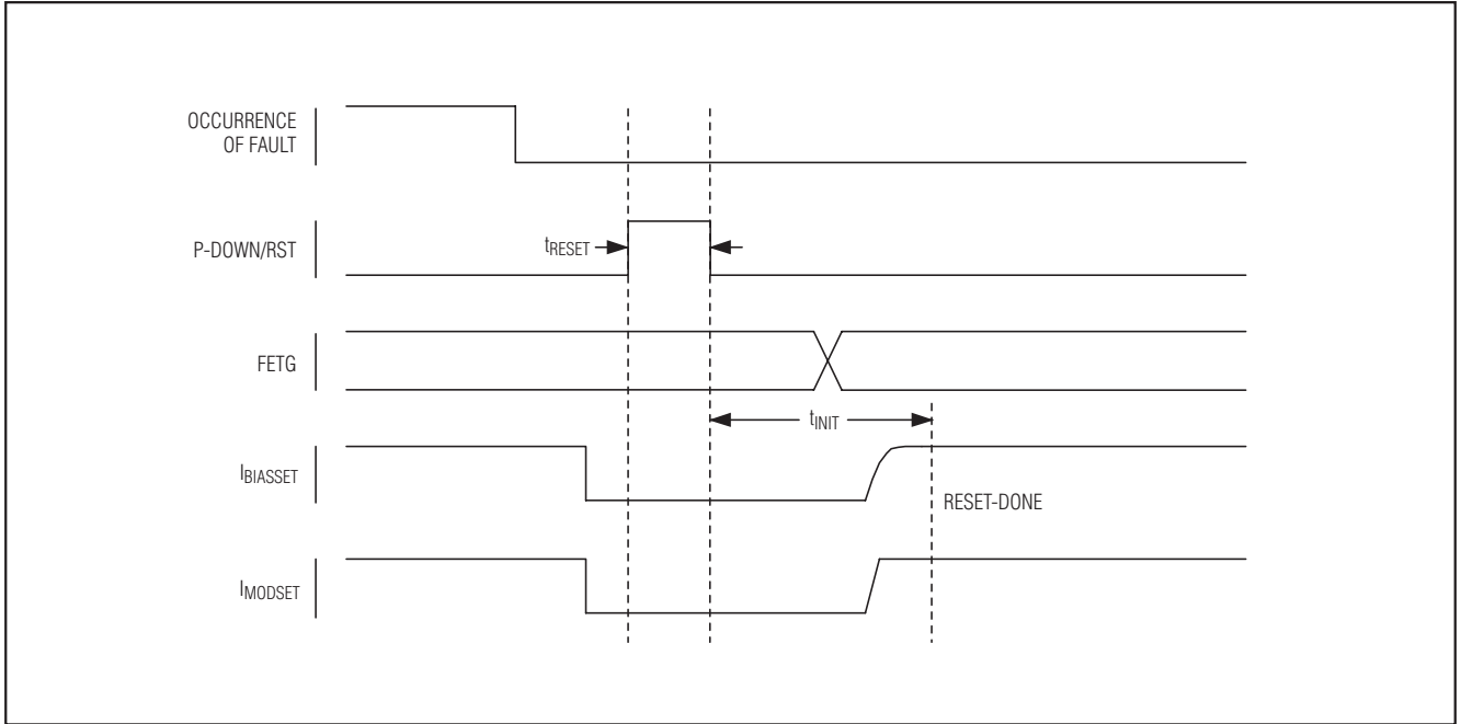
图5. 利用P-DOWN/RST从瞬时故障状态下恢复
