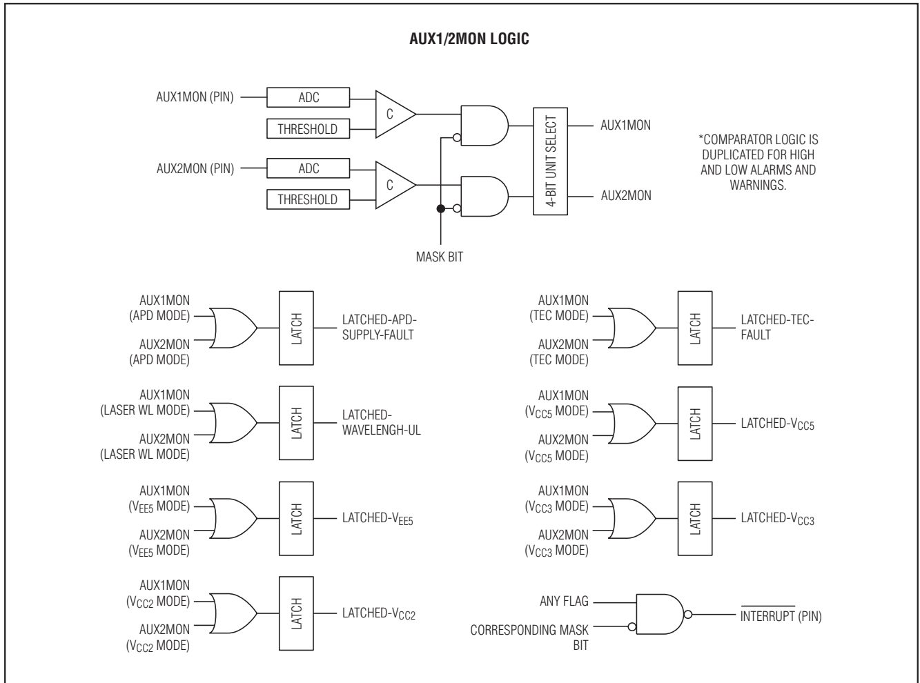
图10. AUX1/2监视逻辑电路
