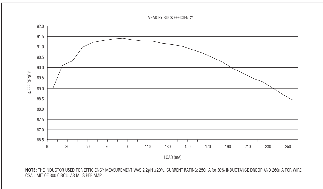
图7a. 使用2.2μH电感时存储器降压稳压器的效率
