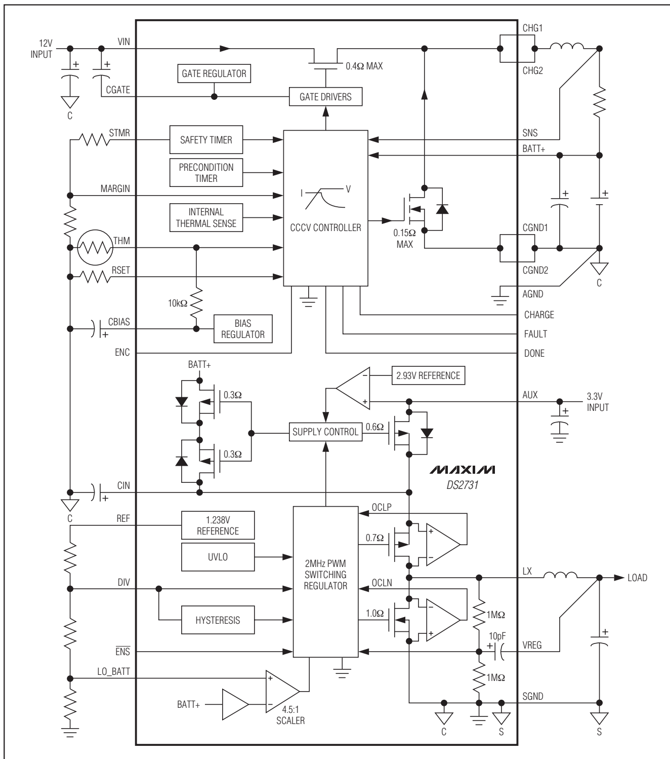
图2. 方框图
