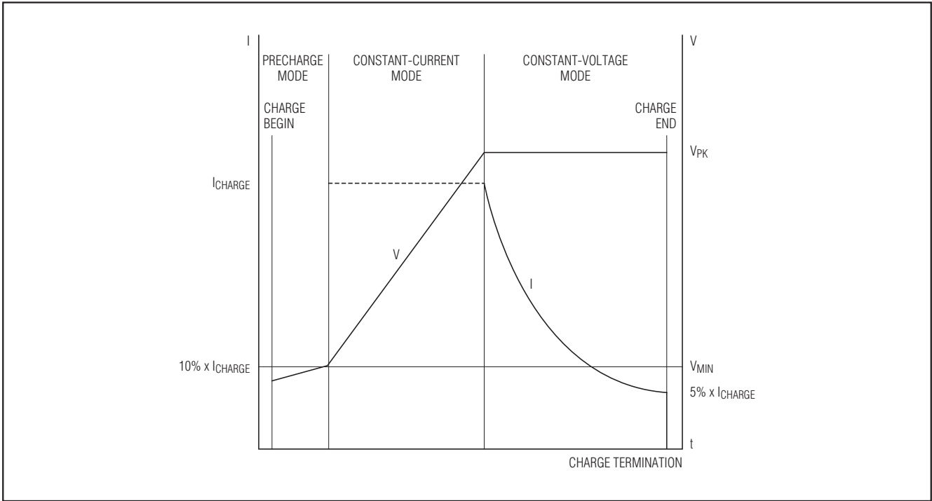
图4. Li+ 电池充电特性
