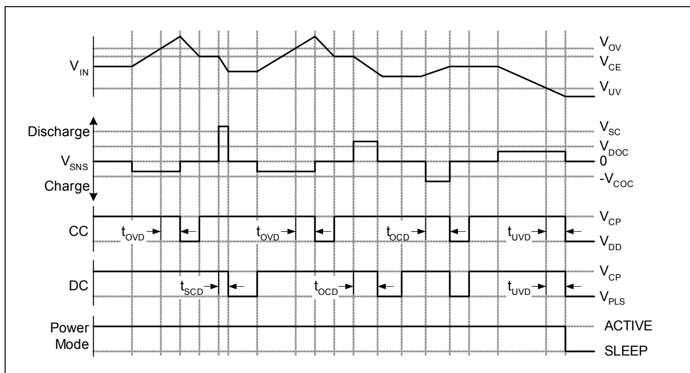
图 2. Li+ 电池保护电路实例波形
