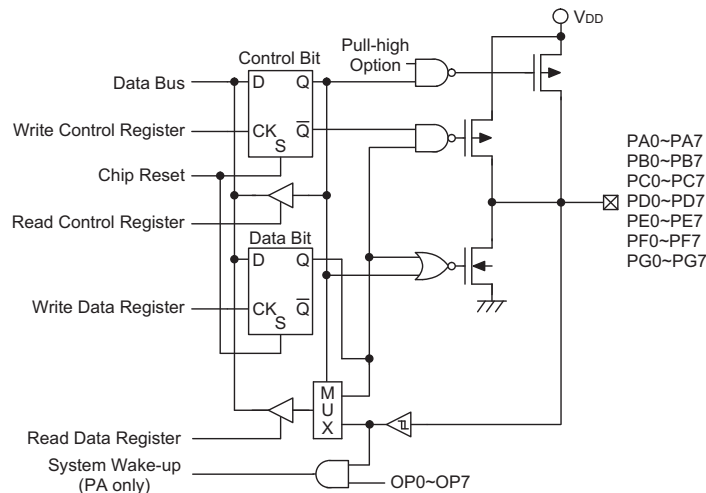
输入/输出
