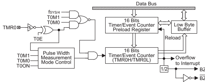
定时/计数器 0
