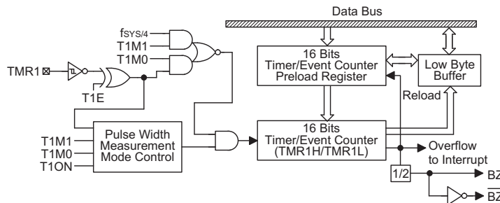
定时/计数器 1
