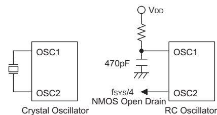
系统振荡器
