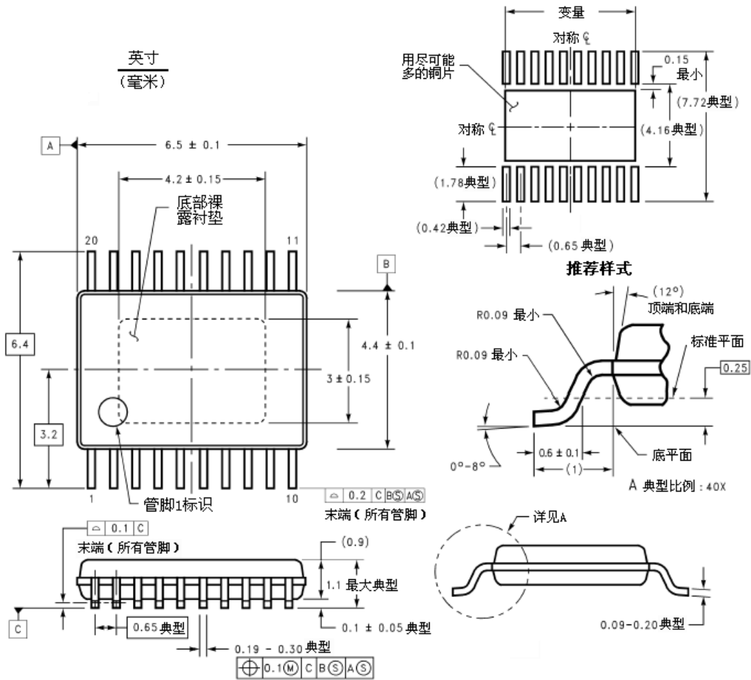
20-引脚模式 TSSOP 封装
