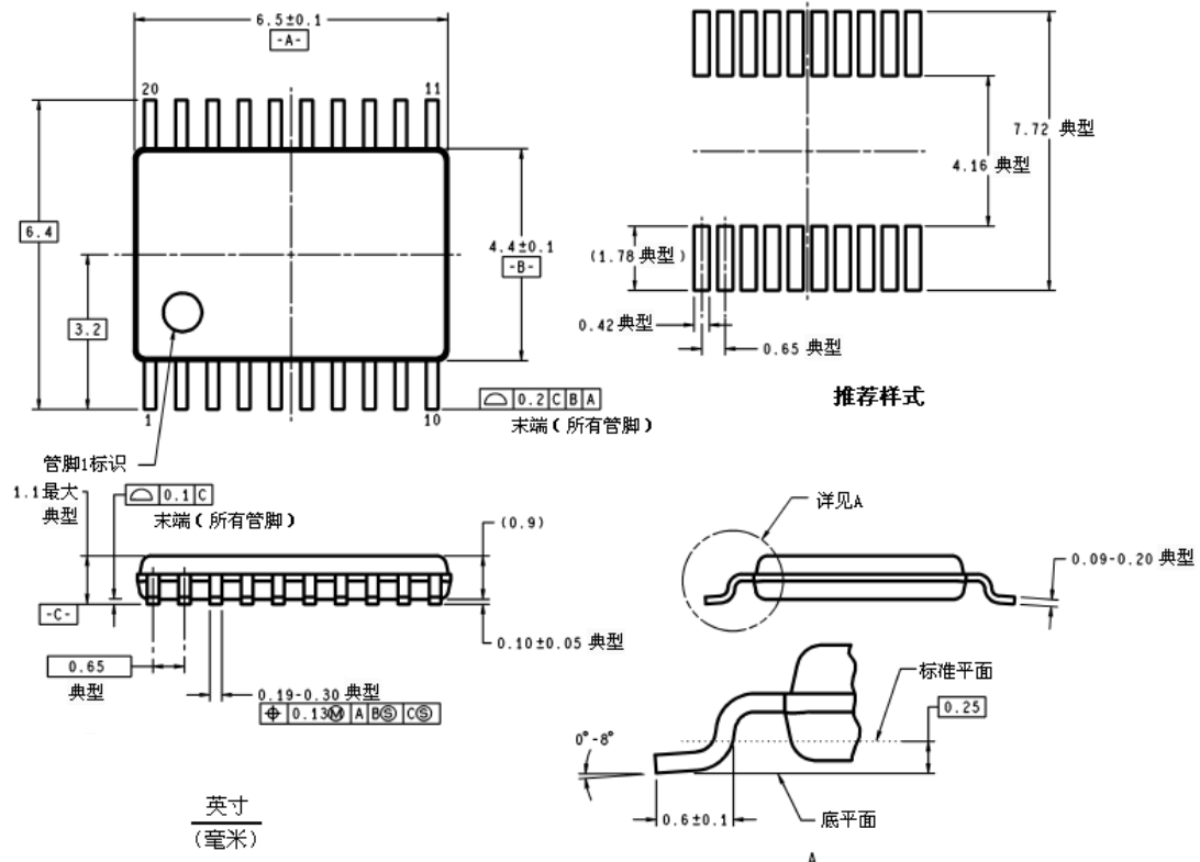
20- 引脚模式 PKG, TSSOP 封装, JEDEC, 主体部分宽 4.4mm
