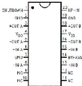
俯视图
