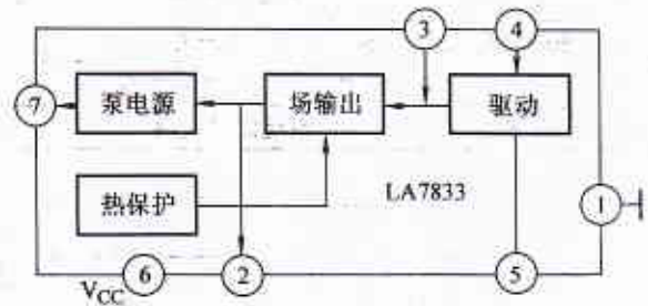
图 265 LA7833 内电路框图
