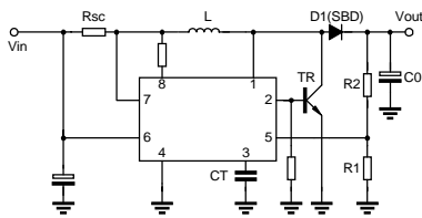
图3 升压变换器 (大电流)
