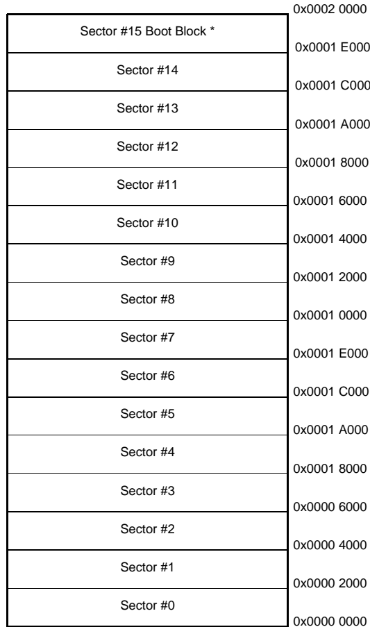
图 34 Flash 扇区映射
