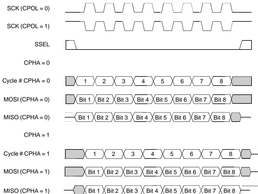
图 24 SPI 数据传输格式 ( CPHA=0 和 CPHA=1 )
