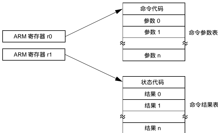
图 37 IAP 参数传递
