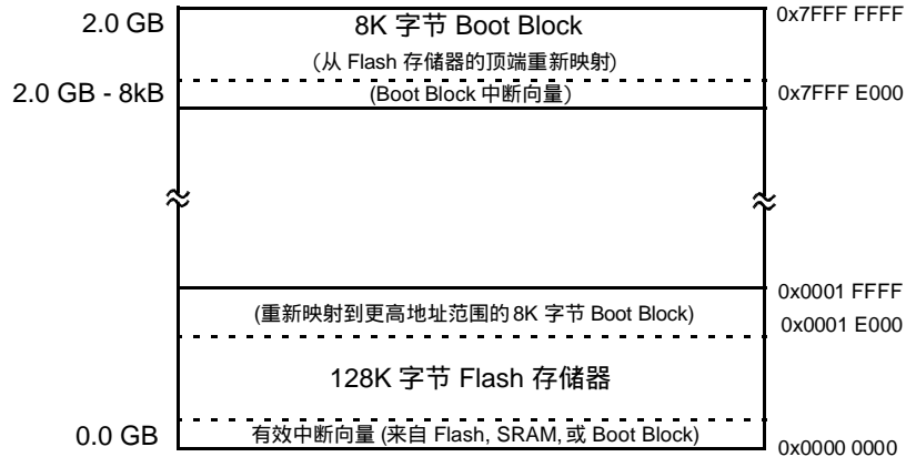
图 35 复位后低地址存储器的映射
