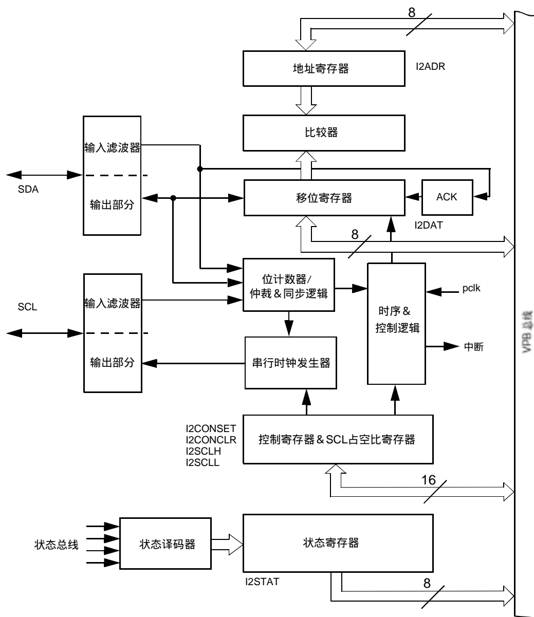
图 23 I 2 C 结构
