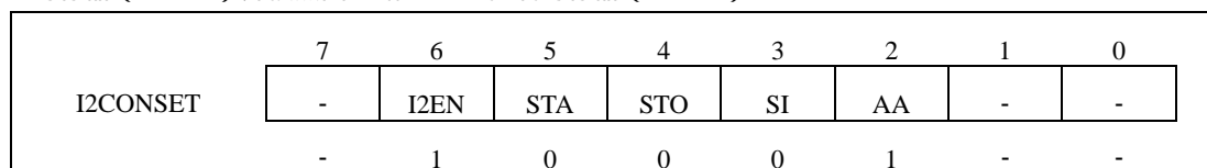
图 20 从模式配置
