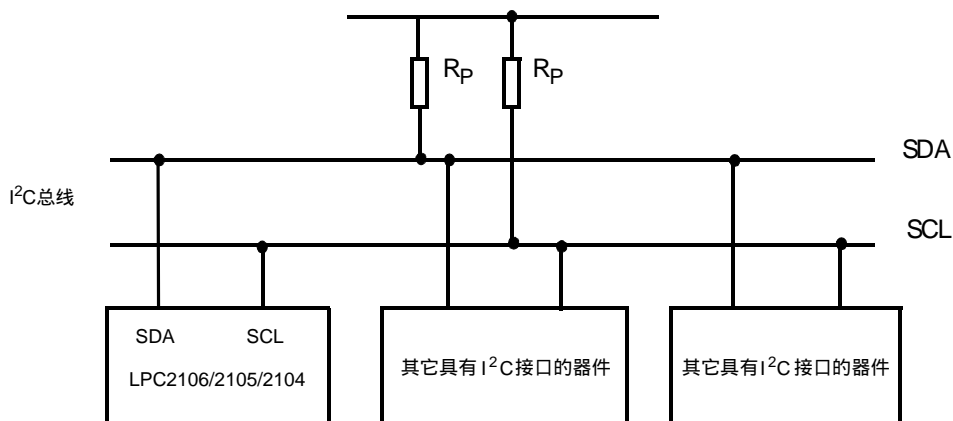
图 15 I 2 C 总线配置
