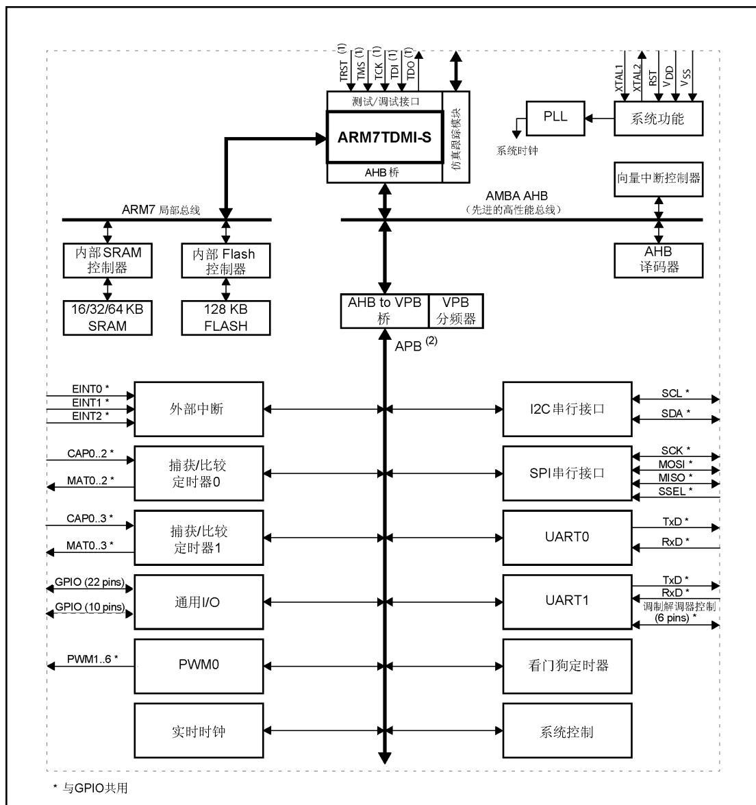
图 1 LPC2106/2105/2104 方框图
