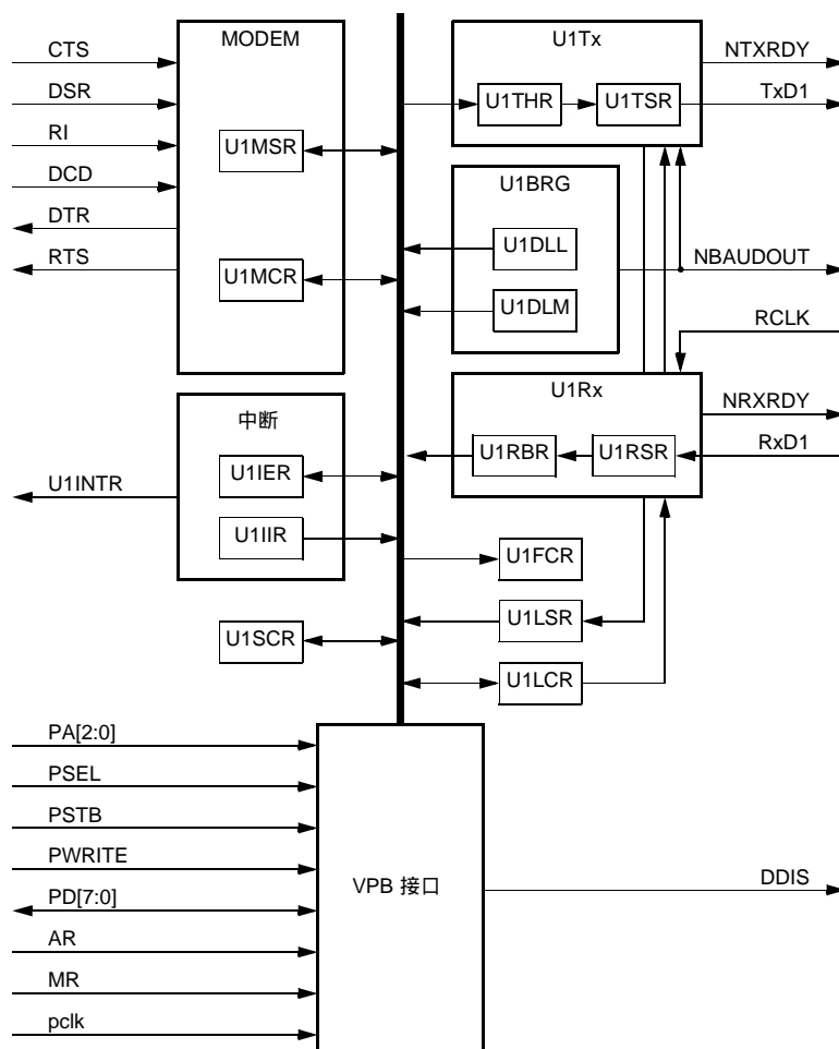
图 14 UART1 方框图
