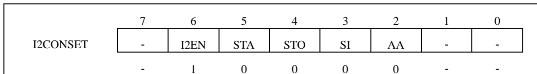
图 16 从模式配置
