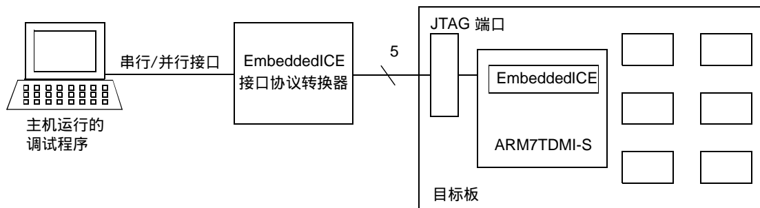
图 38 EmbeddedICE 调试环境方框图
