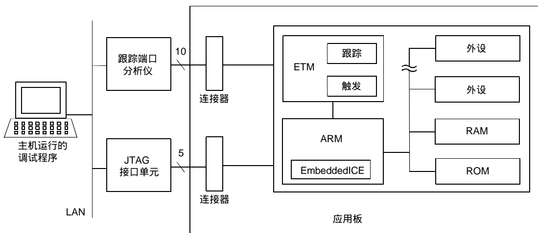
图 41 ETM 调试环境方框图
