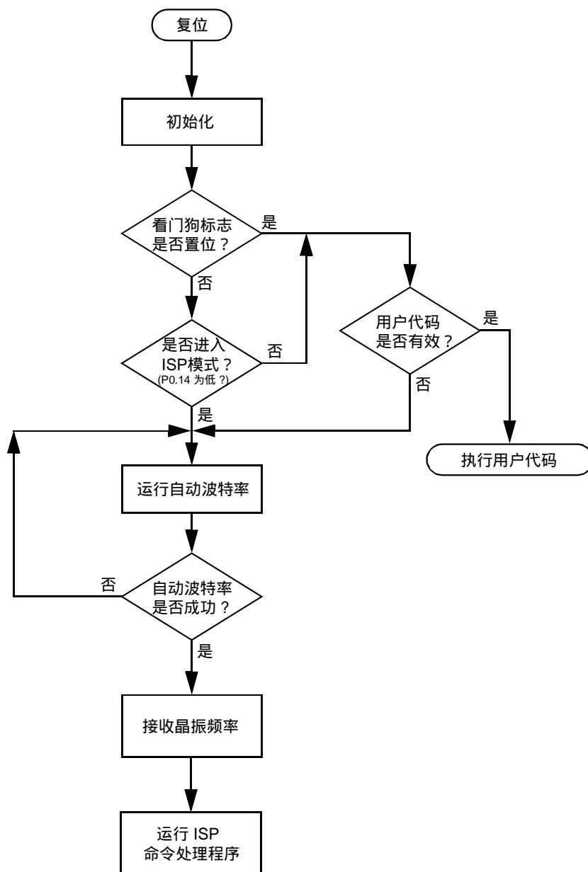
图 36 Boot 处理流程图
