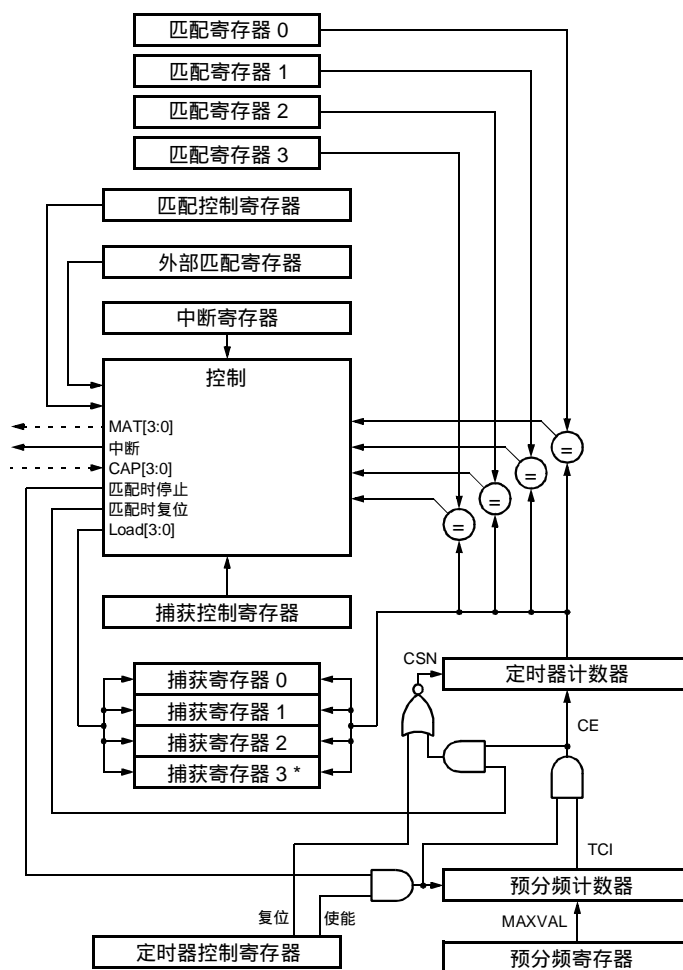
图 28 定时器方框图
