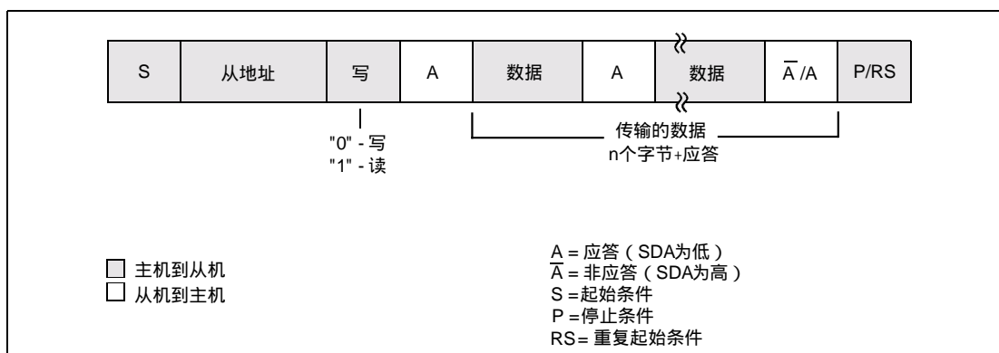
图 21 从接收器模式的格式
