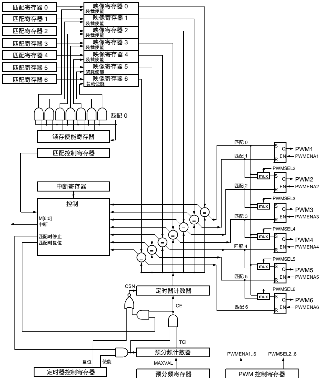
图 29 PWM 方框图
