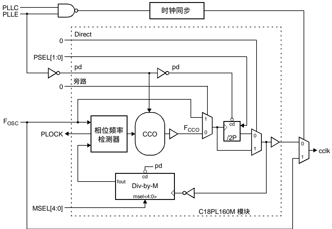
图 8 PLL 方框图
