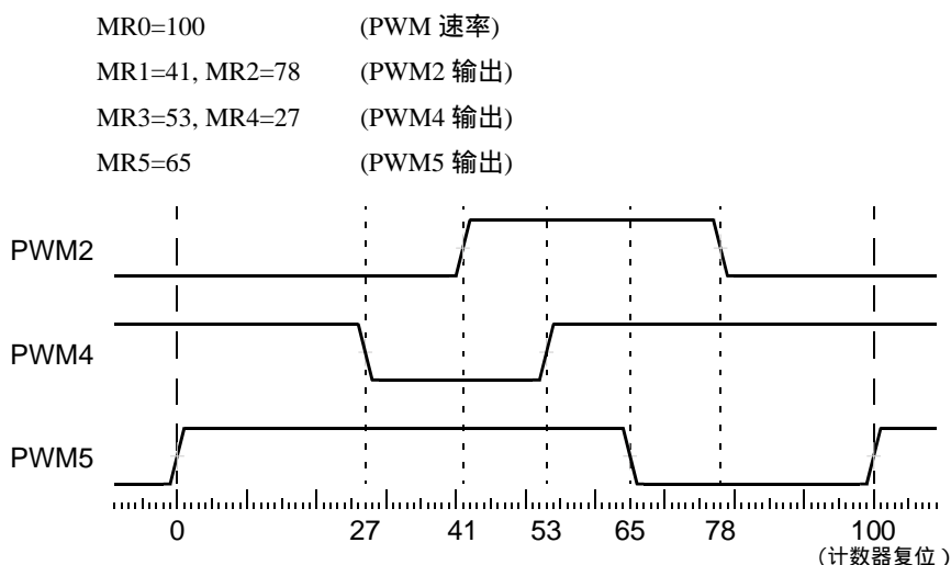
图 30 PWM 波形举例
