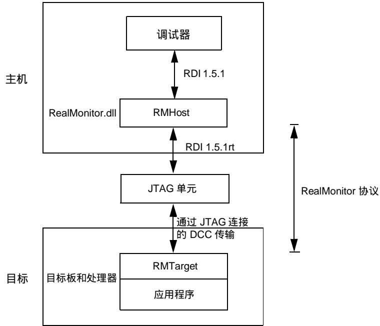
图 42 RealMonitor 部件
