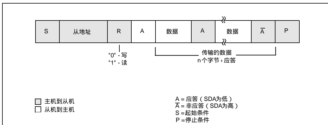
图 22 从发送器模式的格式
