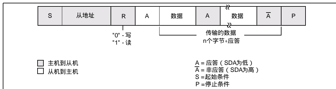
图 18 主接收器模式的格式
