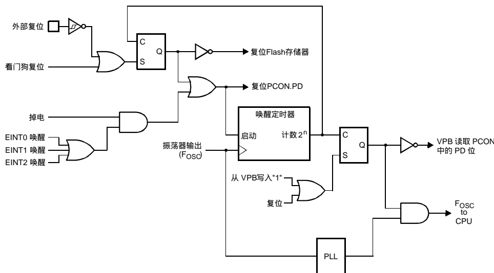
图 9 包括唤醒定时器的复位方框图
