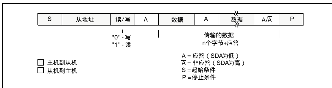
图 17 主发送器模式中的格式
