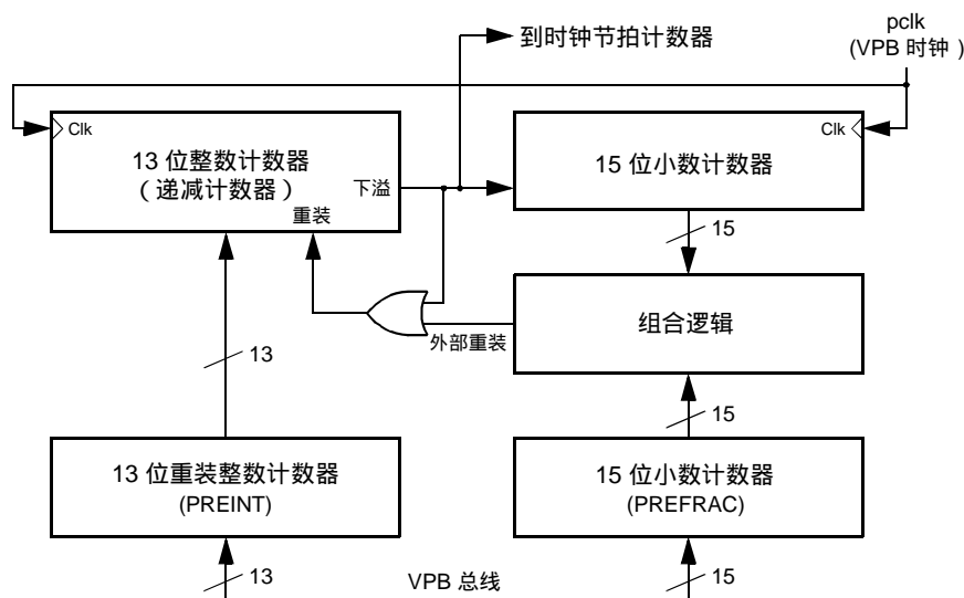
图 32 RTC 预分频器方框图
