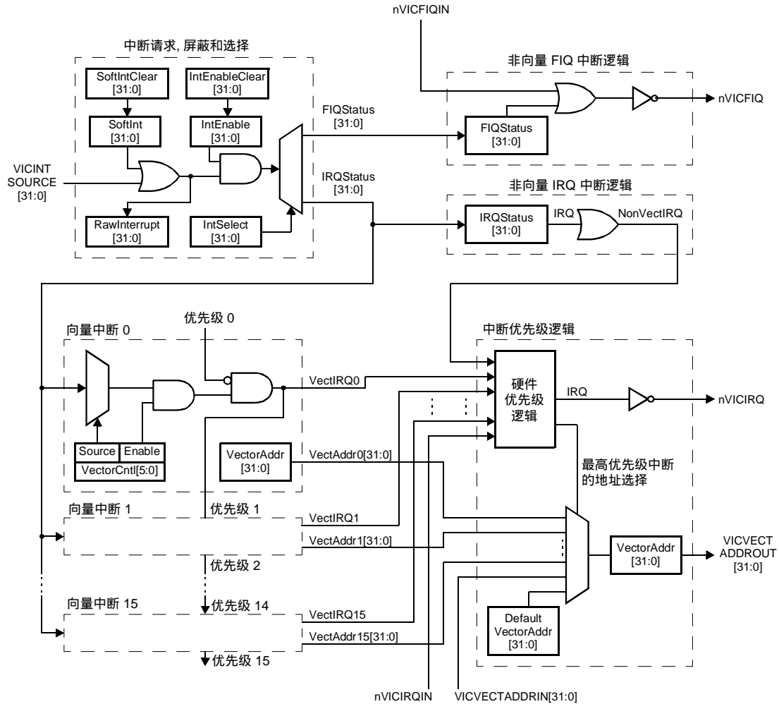
图 12 向量中断控制器方框图
