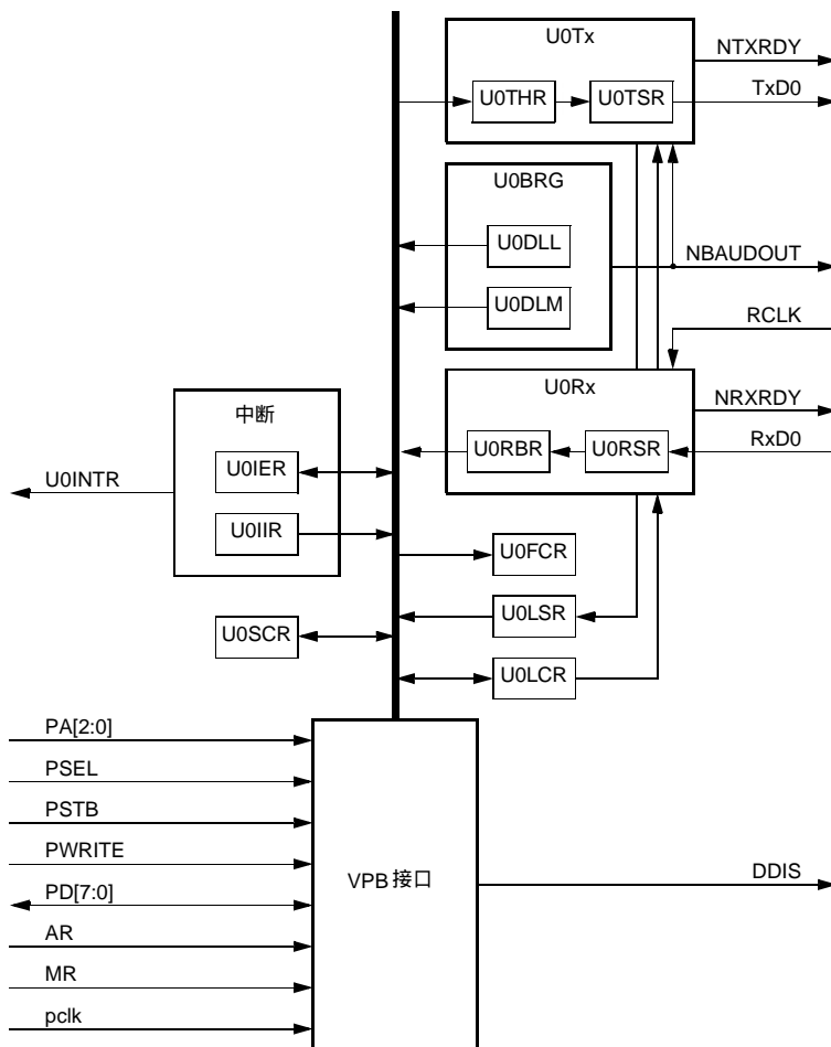
图 13 UART0 方框图
