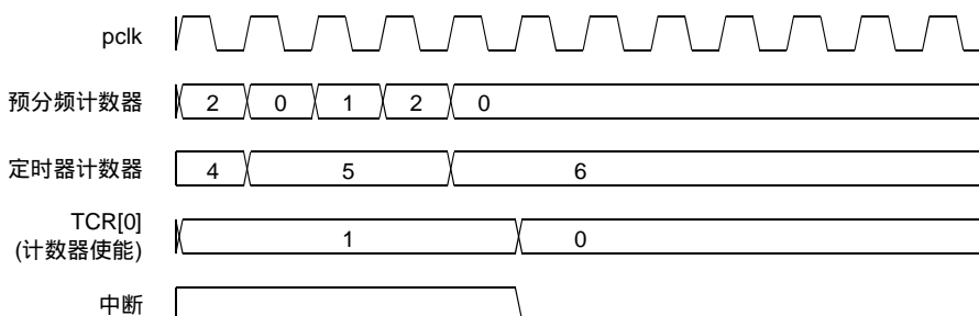
图 27 定时器周期设置为 PR=2, MRx=6, 匹配时使能中断和停止
