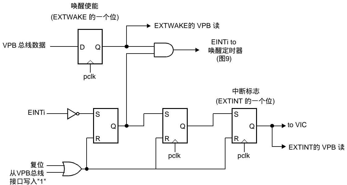
图 7 外部中断逻辑
