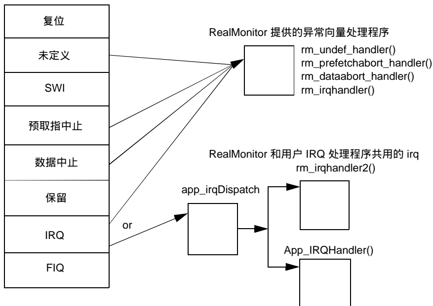
图 44 异常处理程序
