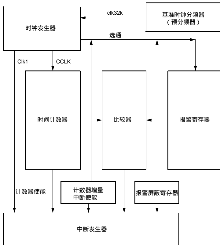
图 31 RTC 方框图
