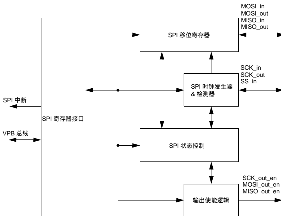
图 25 SPI 方框图
