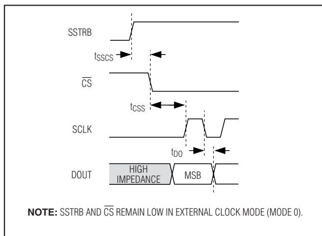
图16. DOUT和SSTRB时
