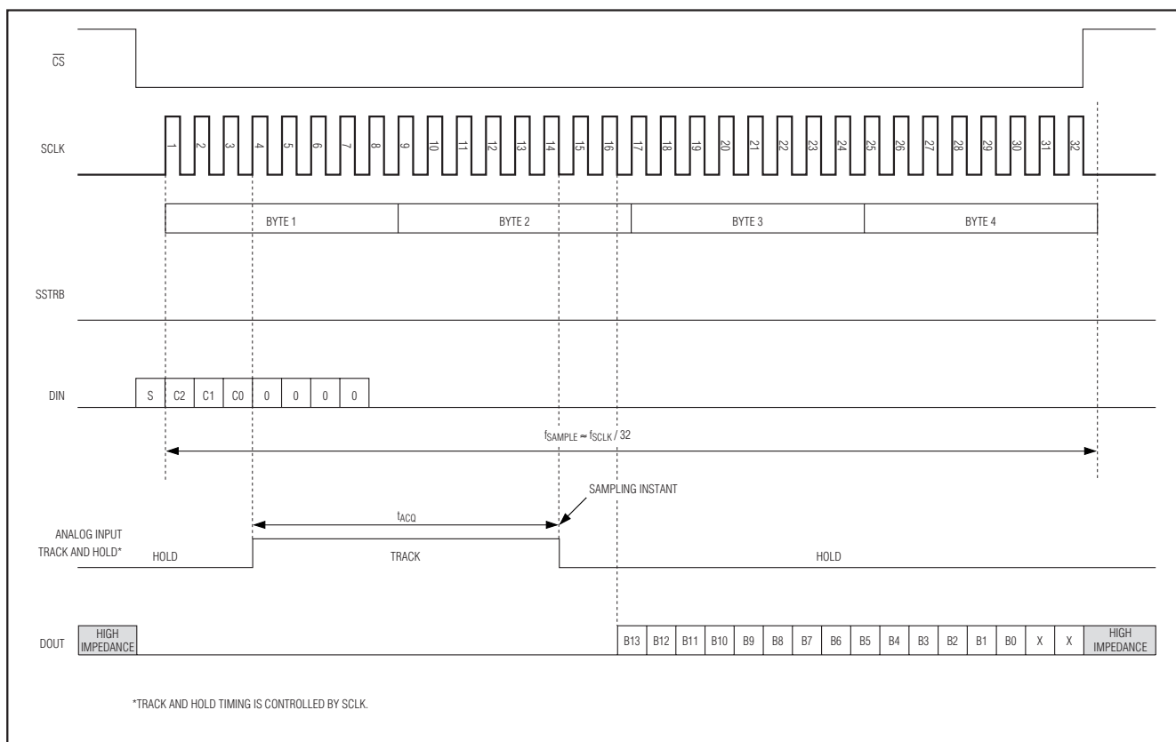
图2. 外部时钟模式 (模式0)
