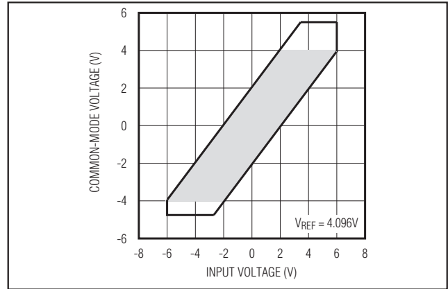
图10. 共模电压与输入电压的关系( FSR = 2 \times V_{REF} )
