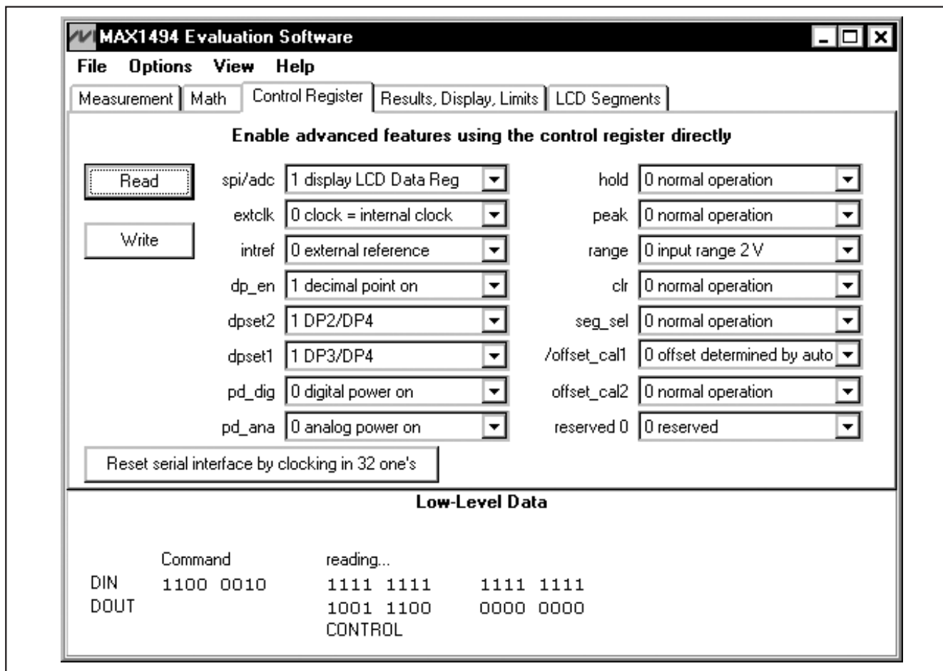
图3. Control Register选项卡页—MAX1494评估软件
