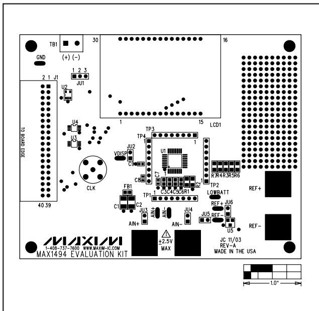
图8. MAX1494 评估板元件摆放指南—顶层丝印层
