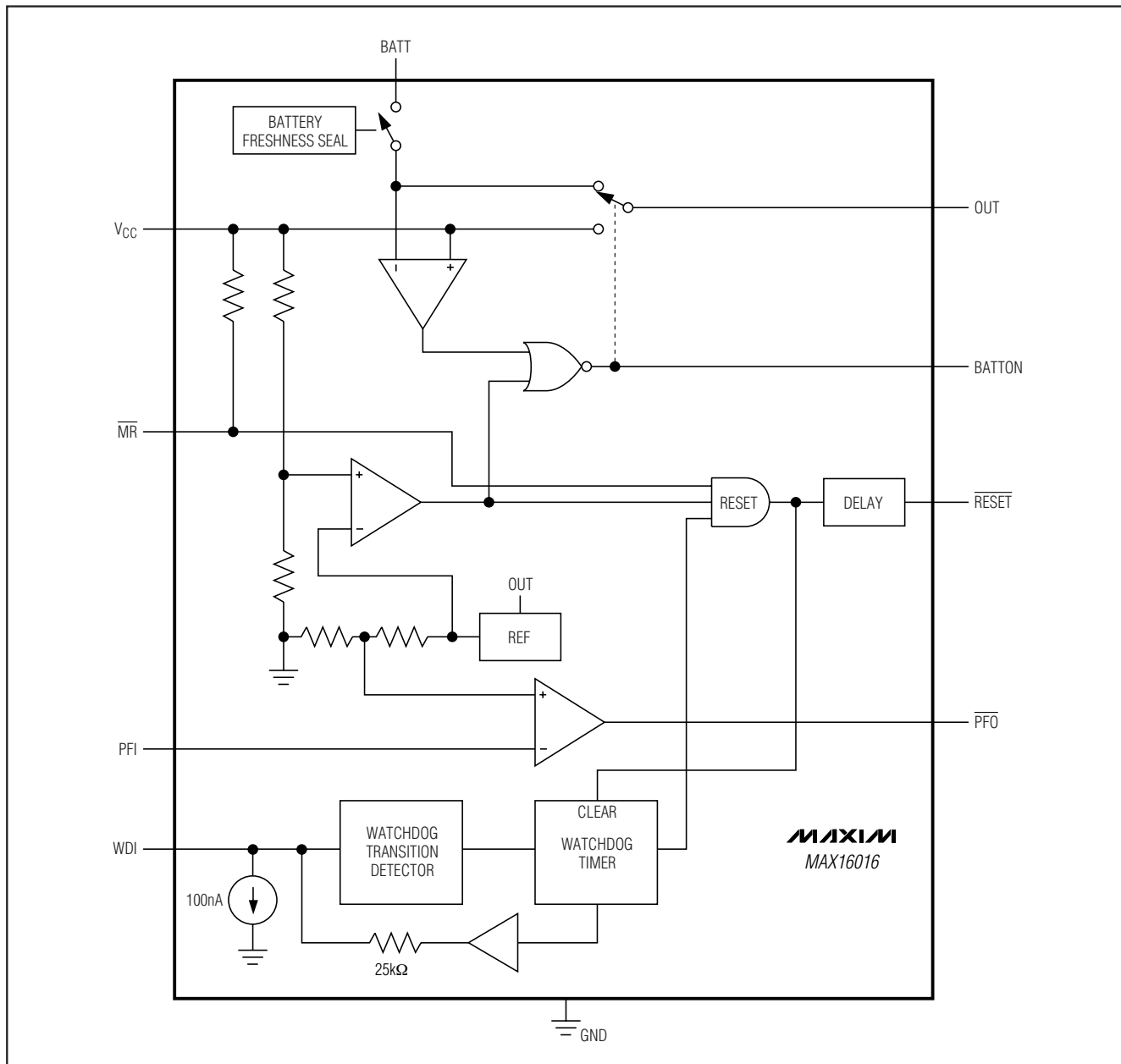
功能框图
