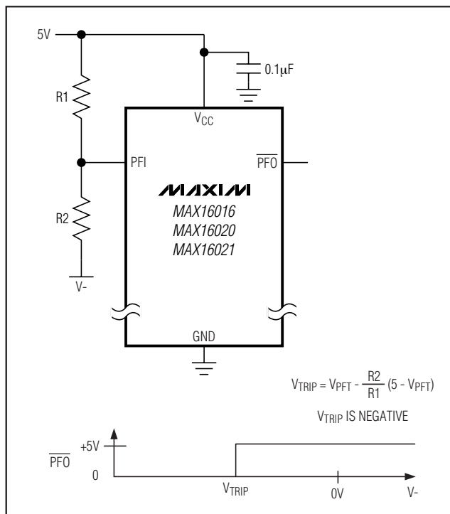
图3. 监测负电源
