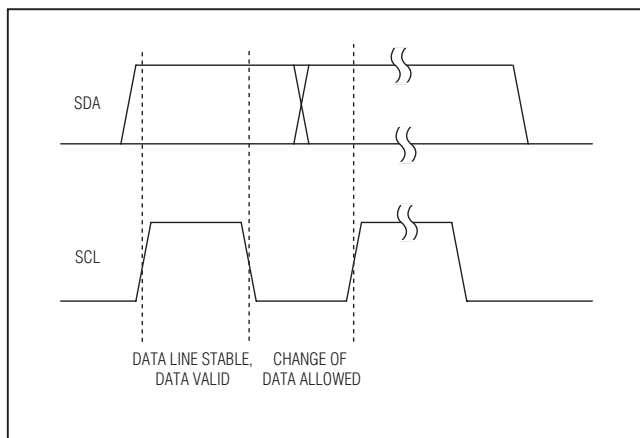
图8. 位传输
