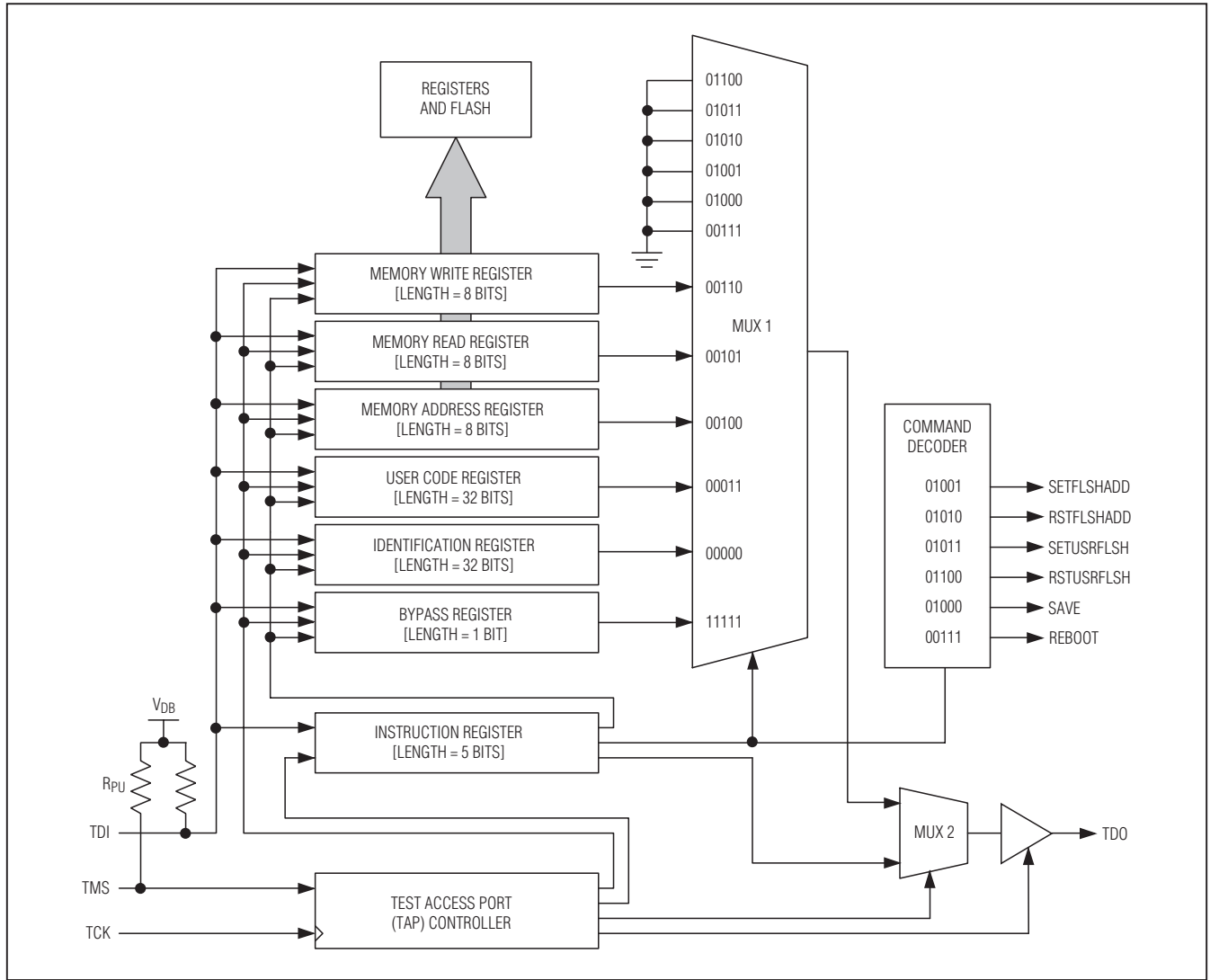
图12. JTAG方框图
