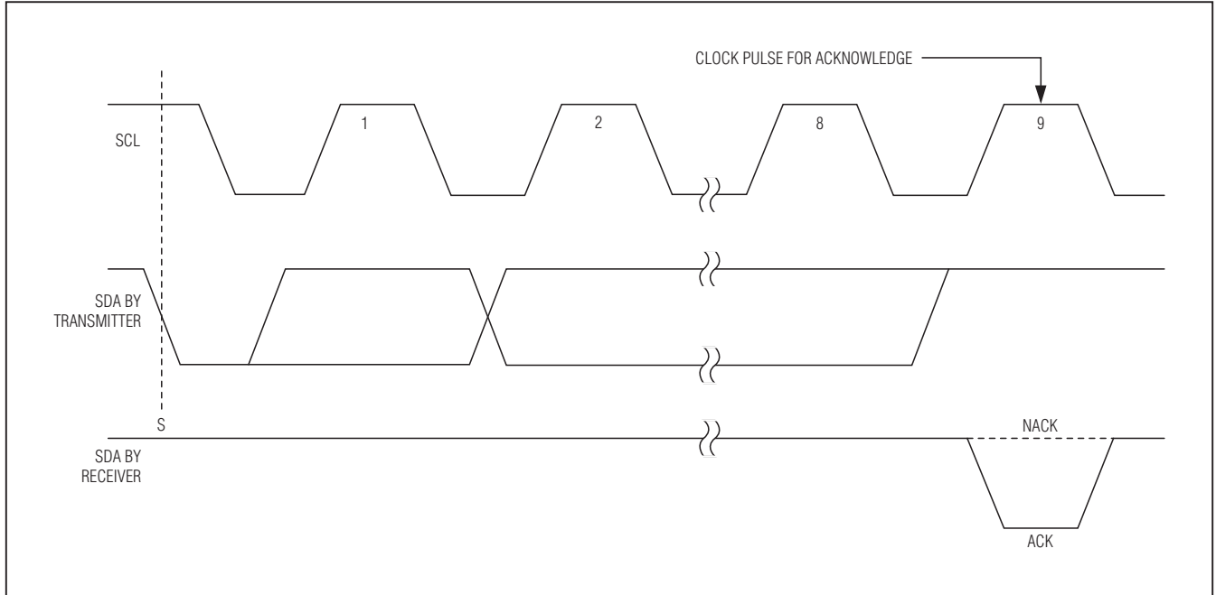
图10. 应答
