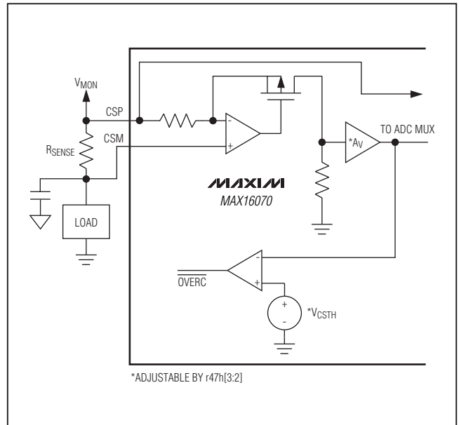
图4. 检流放大器
