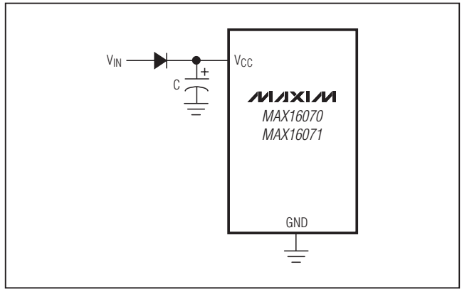
图14. 发生故障期间维持关断状态下的供电电路
