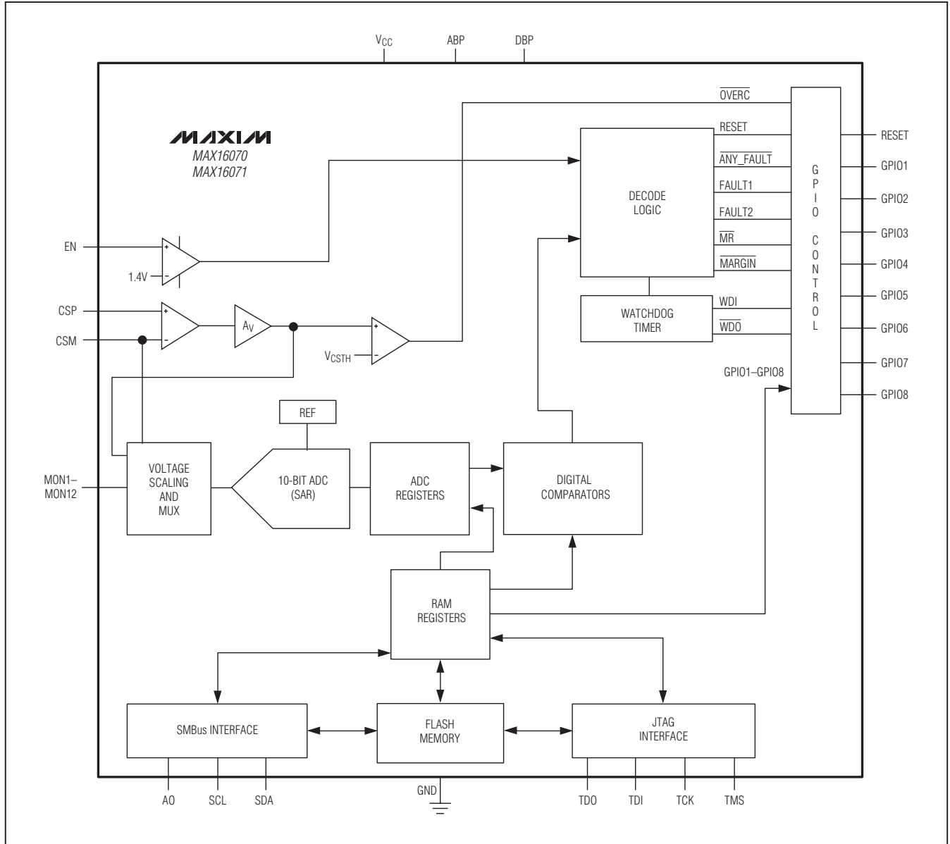
功能框图
