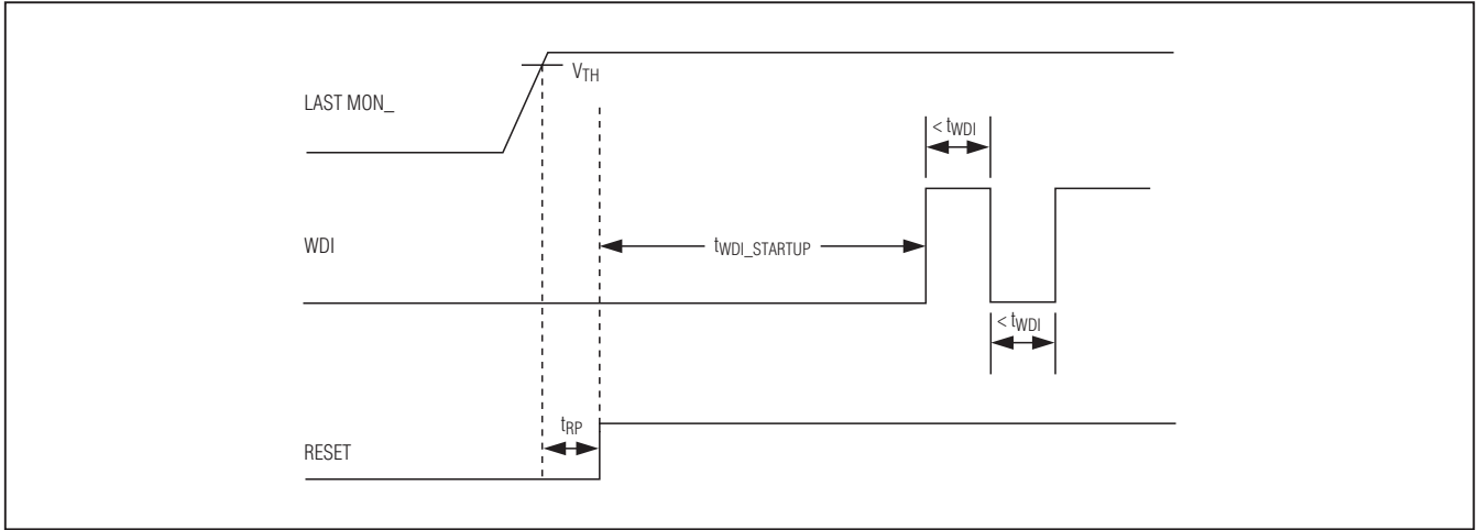
图5. 标准的看门狗启动时序
