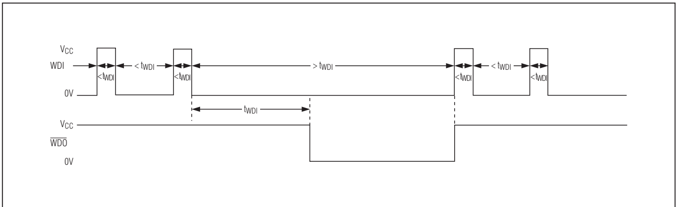
图6. 看门狗定时器工作原理
