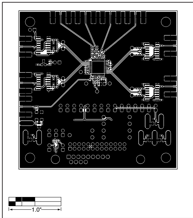
图3. MAX2828/MAX2829 PCB元件层
