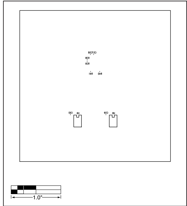
图7. MAX2828/MAX2829 PCB低层丝印图
