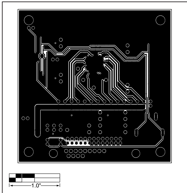
图5. MAX2828/MAX2829 PCB中间第3层
