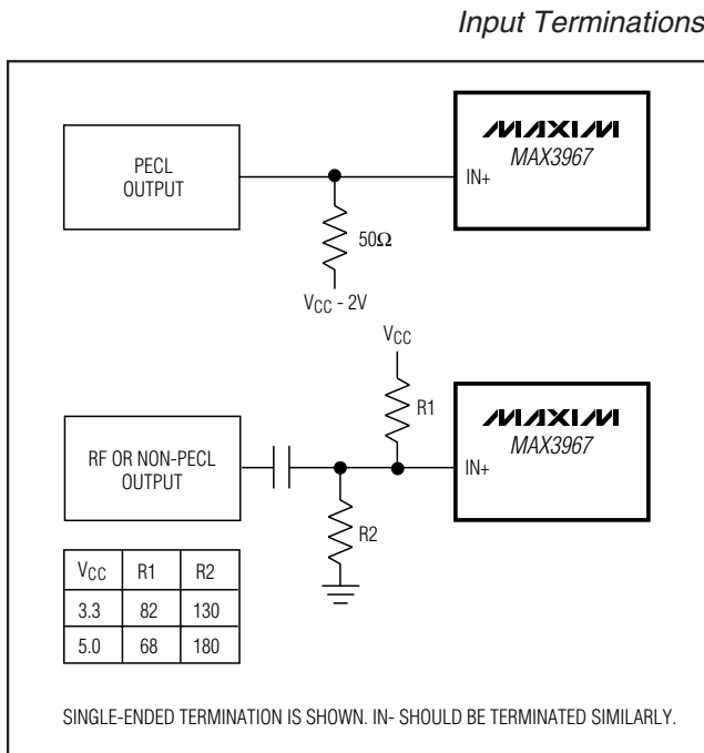
图 3. 输入端接
