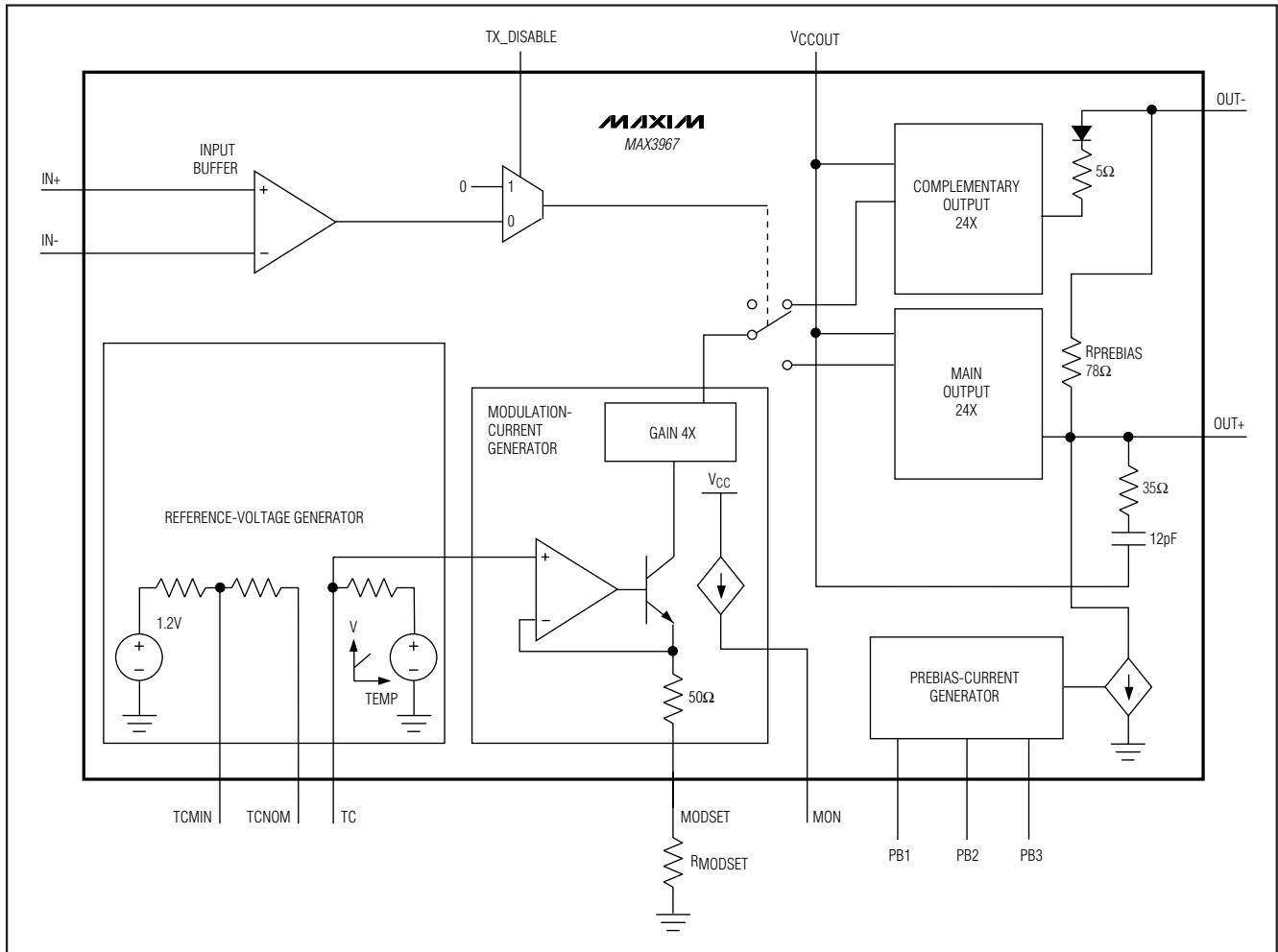
图 2. 功能框图
