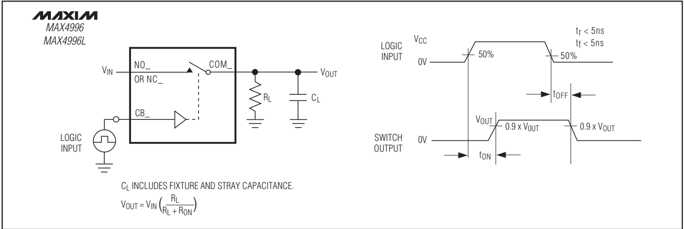
图1. 开关时间
