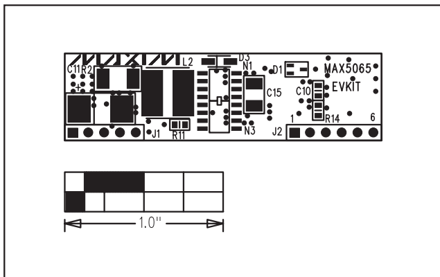
图3. MAX5065 评估板元件布局—顶层
