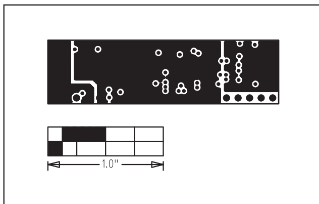
图6. MAX5065 评估板PCB布局—GND, PGND和VOUT (第3层)
