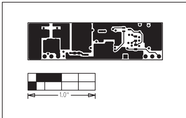
图4. MAX5065 评估板PCB布局—顶层
