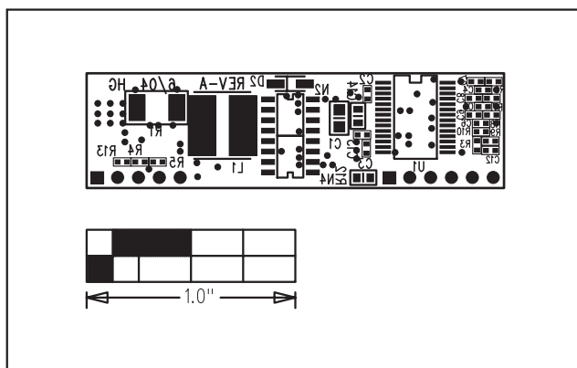
图8. MAX5065 评估板元件布局—底层
