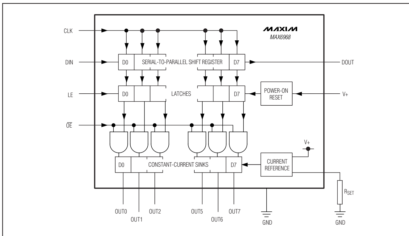
图1. MAX6968方框图
