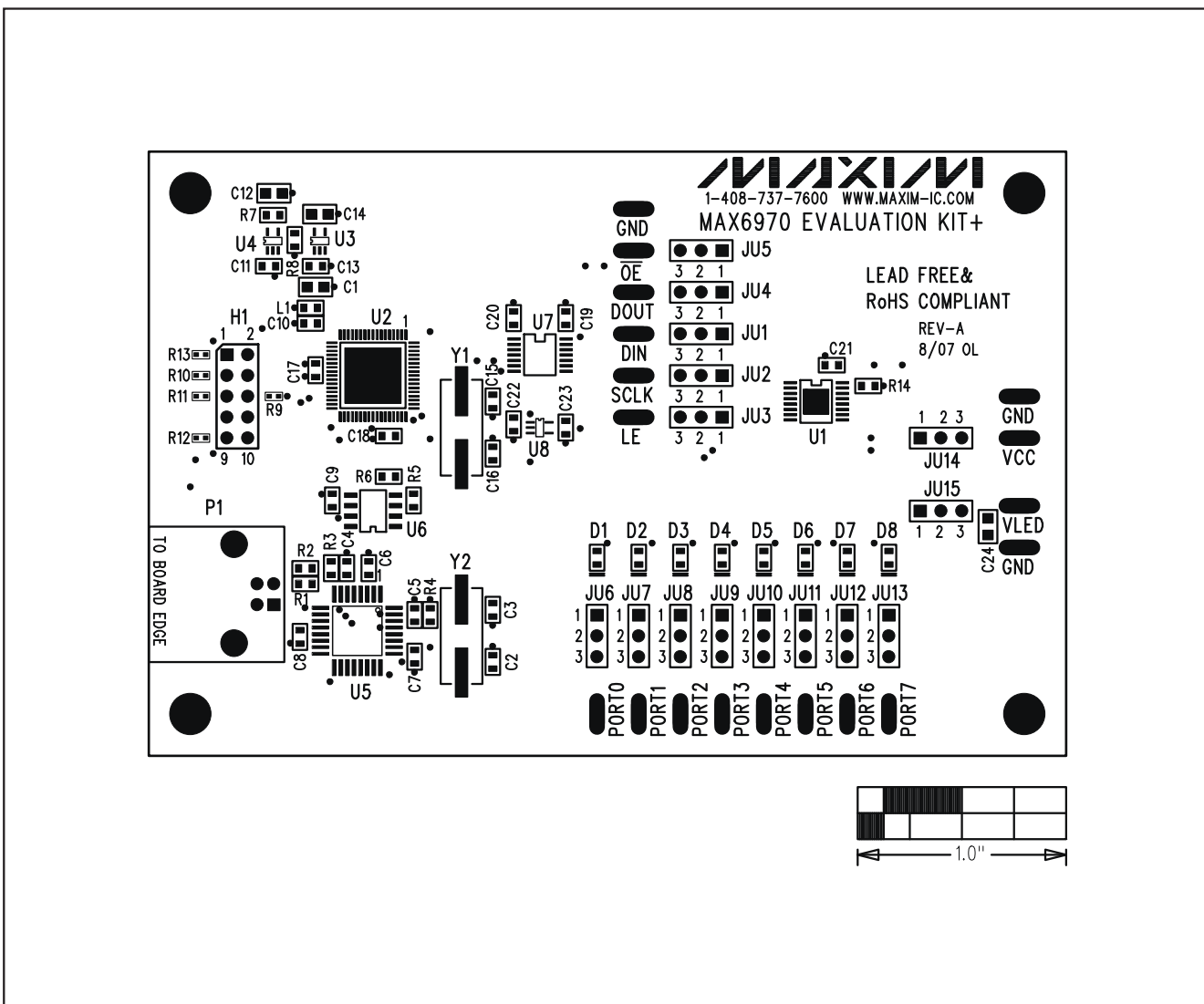
图4. MAX6970评估板元件布局—元件层
