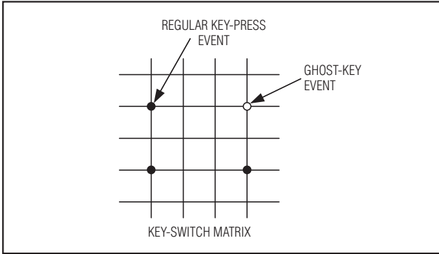
图10. 伪按键操作现象
