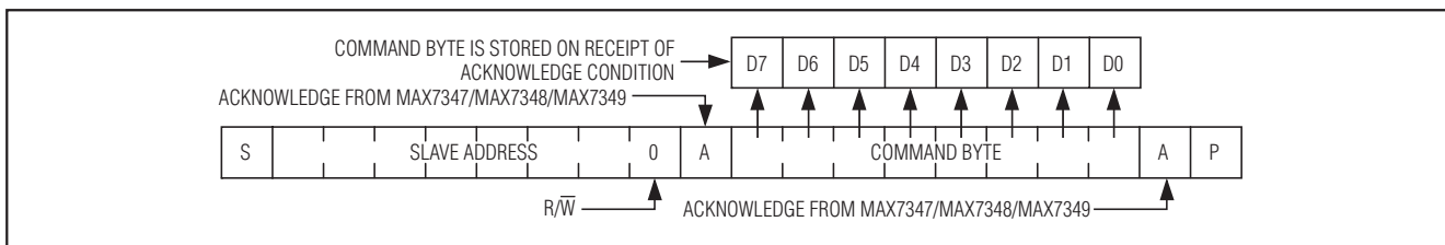
图7. 接收命令字节
