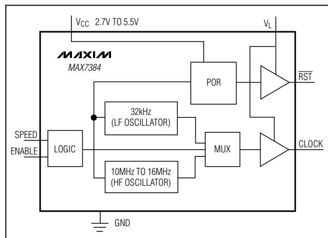
图1. 功能框图
