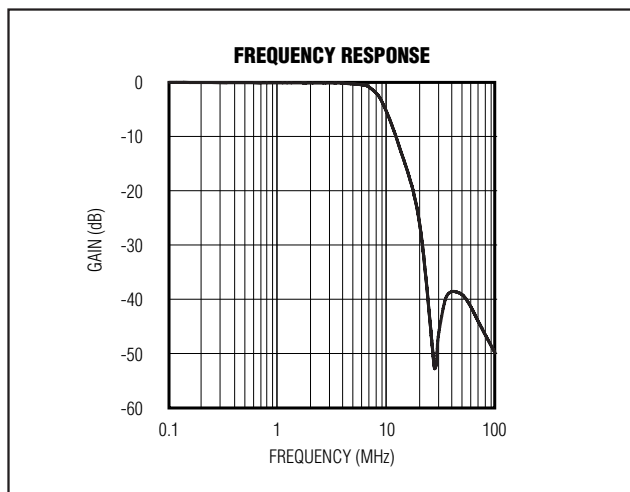
图6. 3阶低通滤波器频率响应
