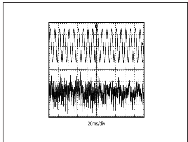
图5. 正弦波与音频信号的RMS比较
