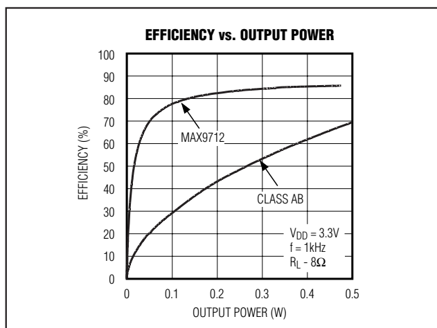
图 5. MAX9712 的效率与 AB 类效率的比较
