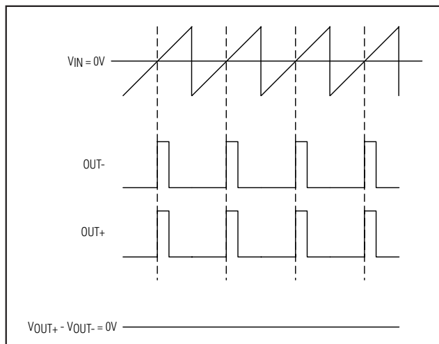
图 4. 无输入信号时 MAX9712 的输出
