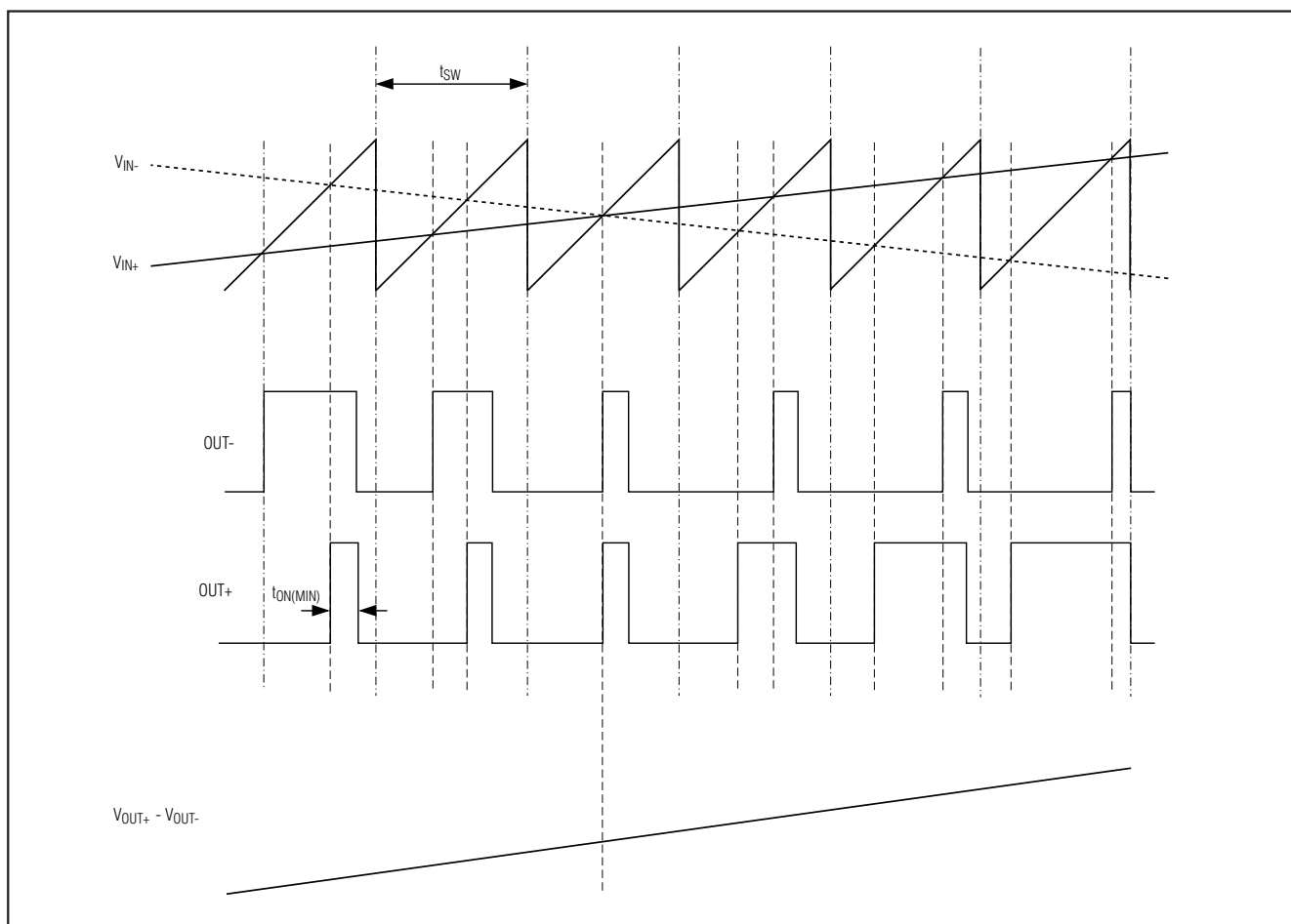
图 1. MAX9712 输出与输入信号的对应关系
