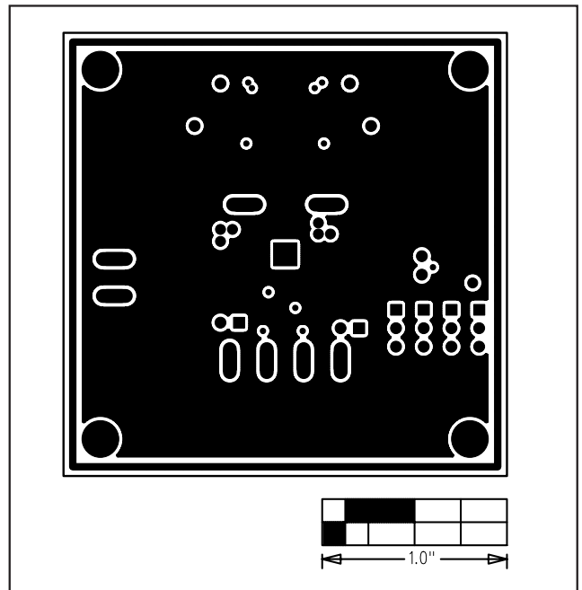
图5. MAX9713评估板PCB布局—第3层(VDD)
