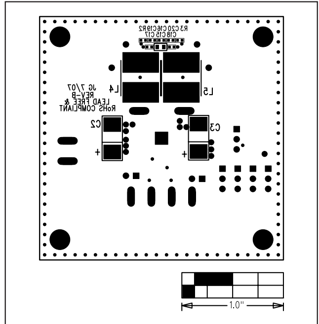
图7. MAX9713评估板元件布局—焊接层
