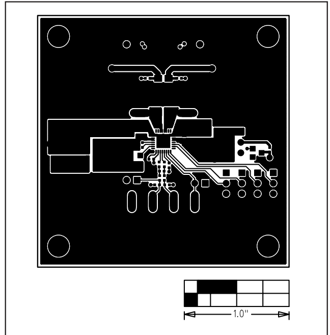
图3. MAX9713评估板PCB布局—元件层
