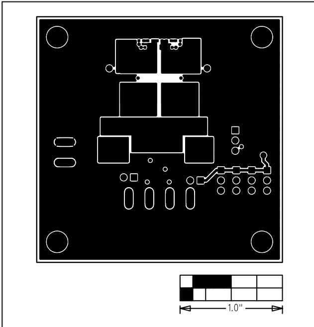
图6. MAX9713评估板PCB布局—焊接层
