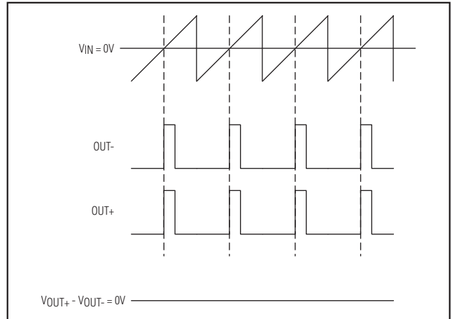
图2. 无输入信号时的MAX9715输出
