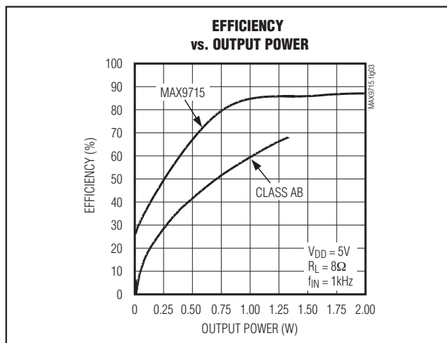
图3. MAX9715 D类放大器与AB类放大器的效率比较
