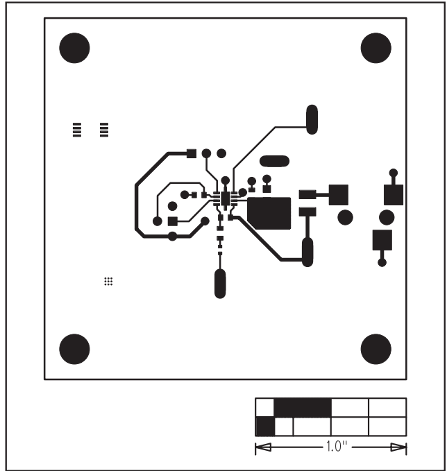
图3. MAX9716 评估板电路板布线——元件层
