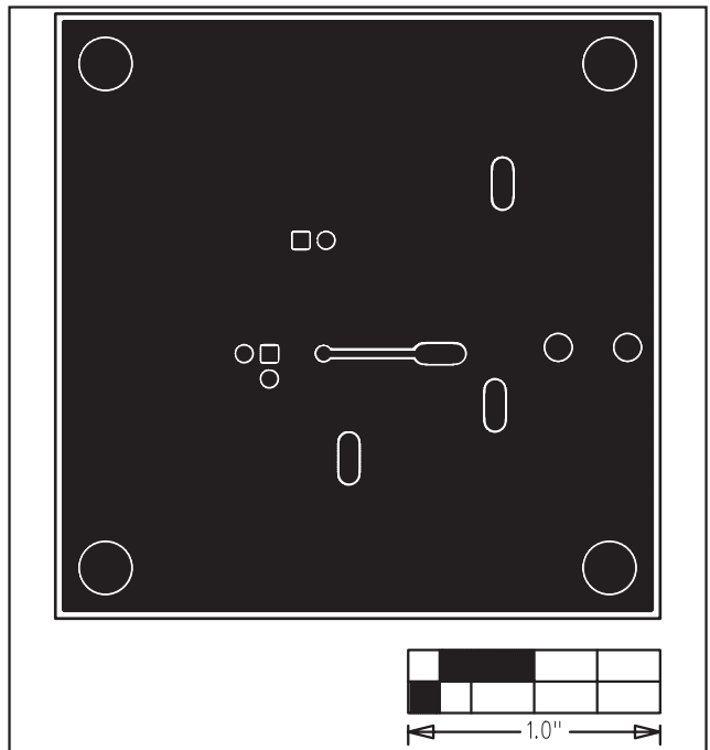
图4. MAX9716 评估板电路板布线——焊接层
