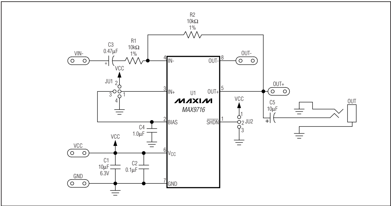
图1. MAX9716评估板原理图
