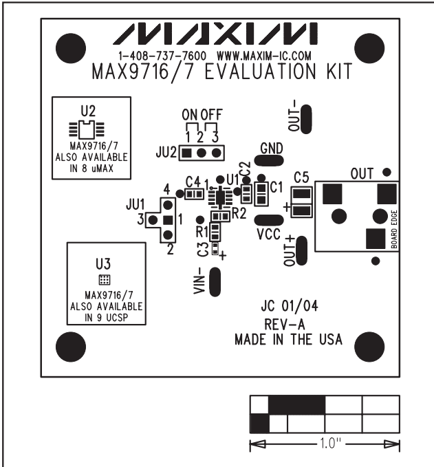
图2. MAX9716 评估板元件摆放指南——元件
