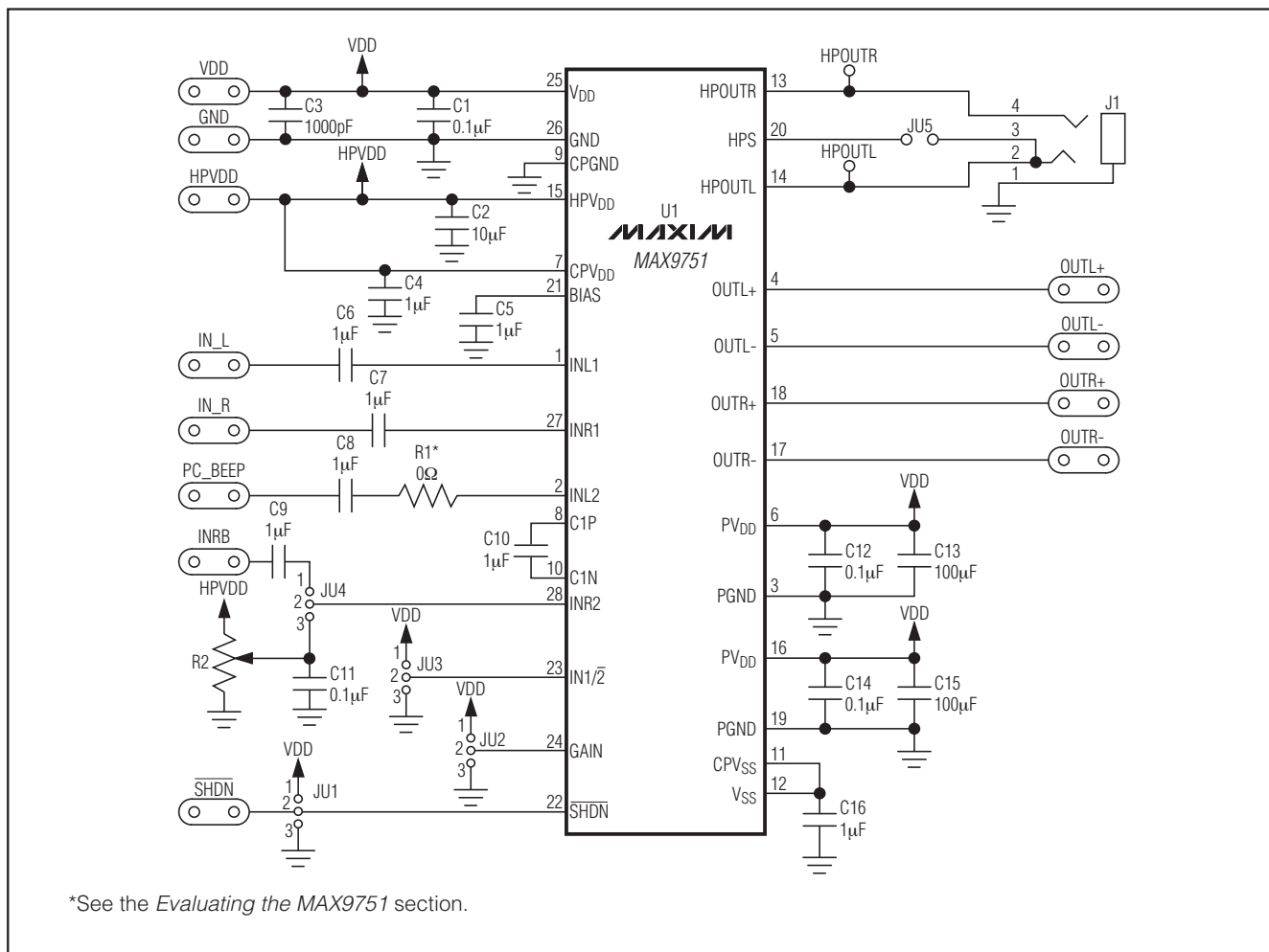
图2. MAX9751 应用电路
