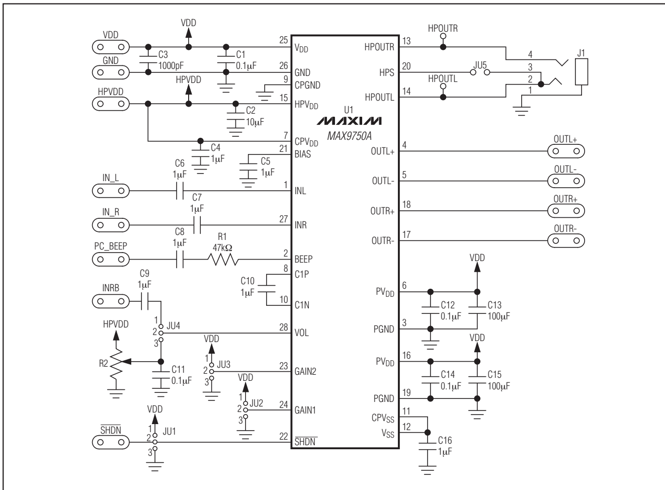
图1. MAX9750A 评估板原理图
