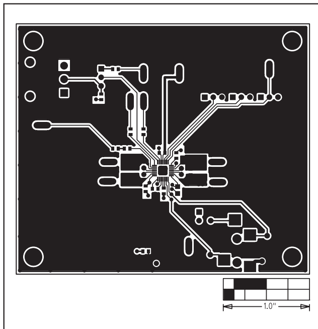
图5. MAX9750A 评估板PCB布局—元件层
