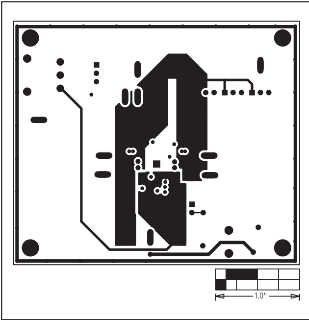
图7. MAX9750A 评估板PCB布局—VDD第3层
