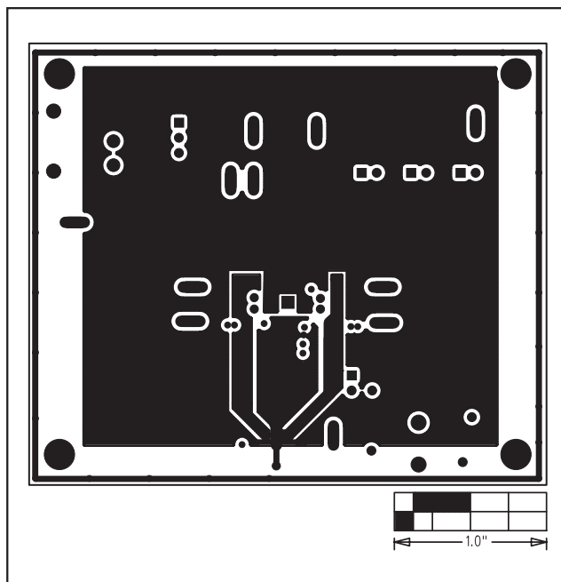
图6. MAX9750A 评估板PCB布局—GND第2层
