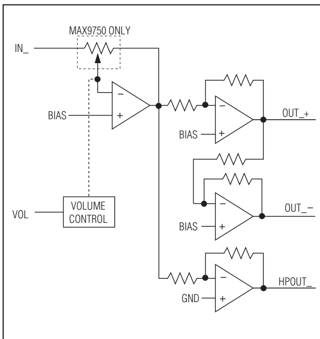
图1. MAX9750/MAX9751信号通道
