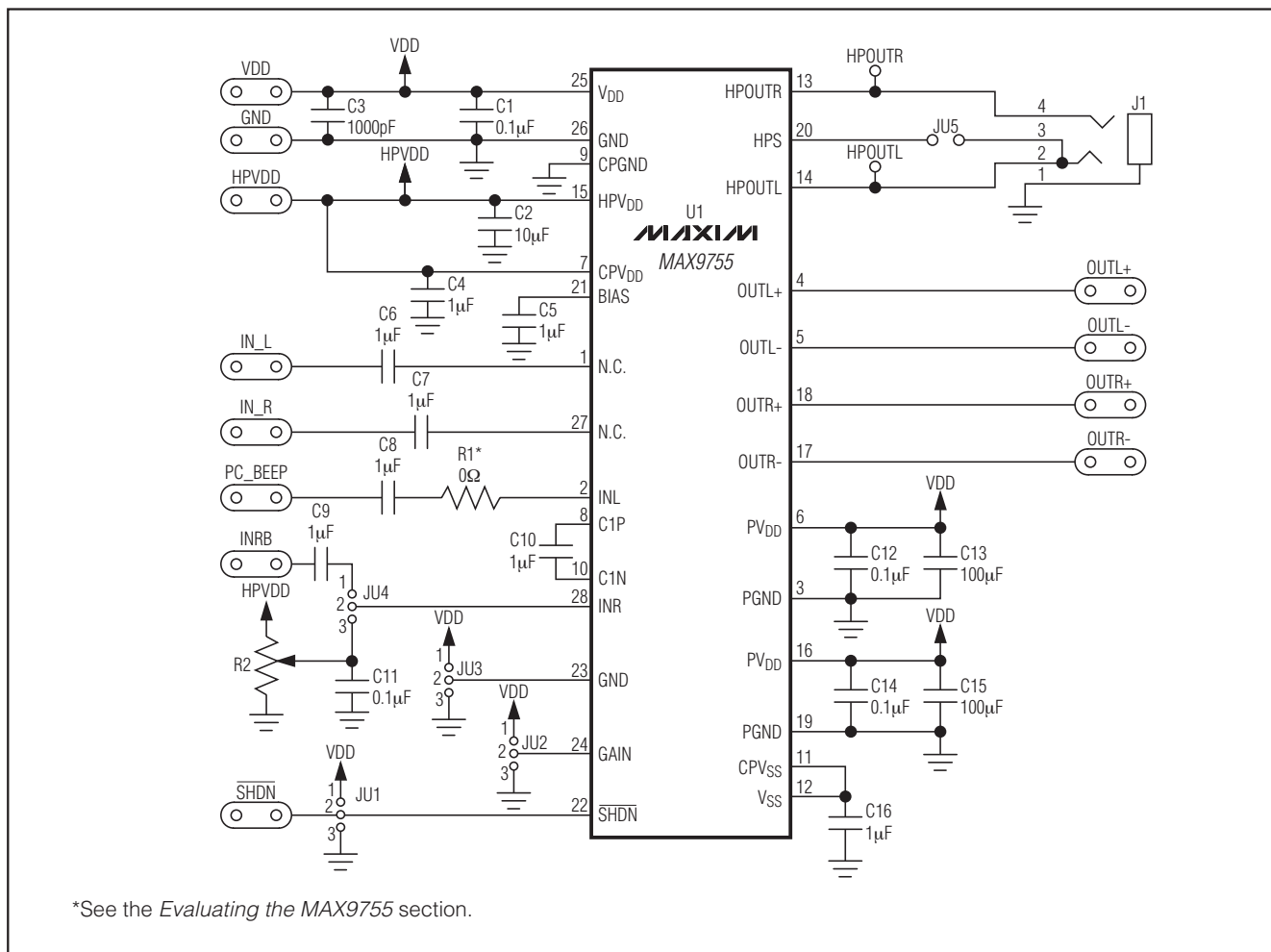
图3. MAX9755 应用电路
