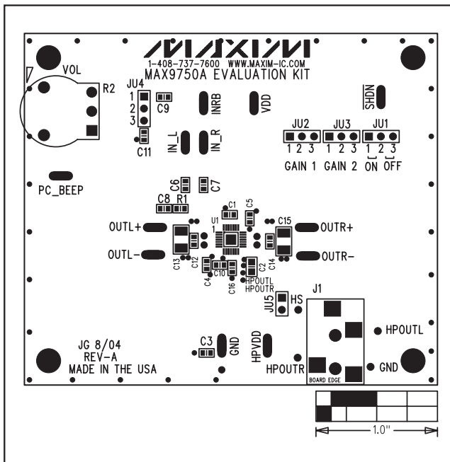
图4. MAX9750A 评估板元件布局—元件层
