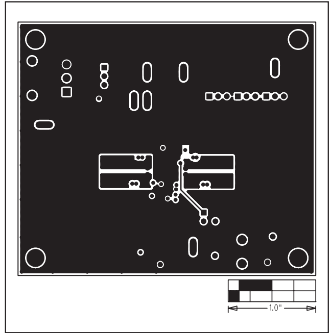
图8. MAX9750A 评估板PCB布局—焊接层
