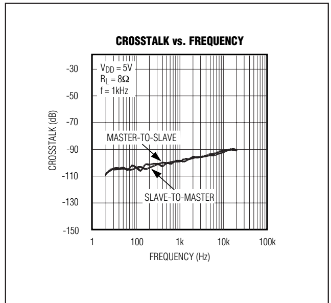
图4. 主-从串扰
