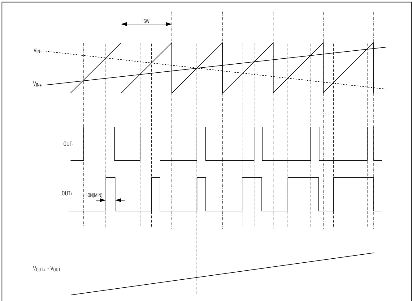
图1. 输入单路信号时 MAX9770/MAX9772 的输出
