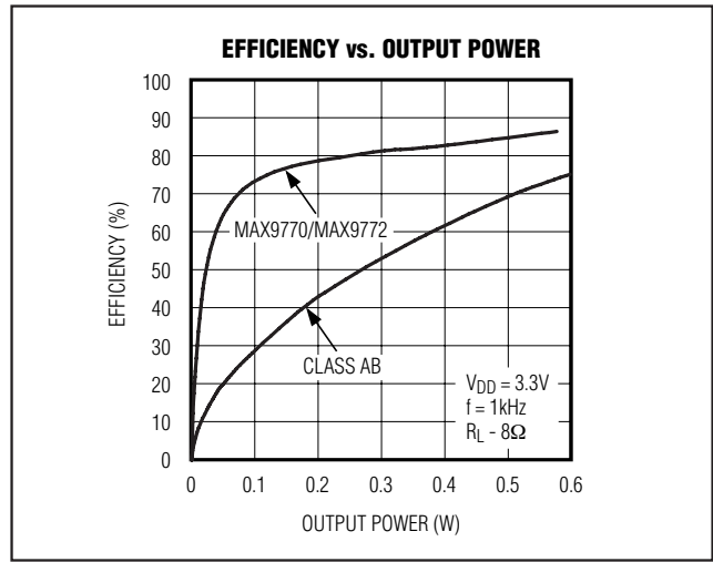
图5. MAX9770/MAX9772 效率与 AB 类效率
