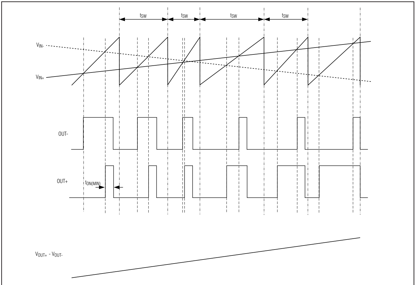
图2. 输入单路信号时 MAX9770/MAX9772 的输出(SSM 模式)
