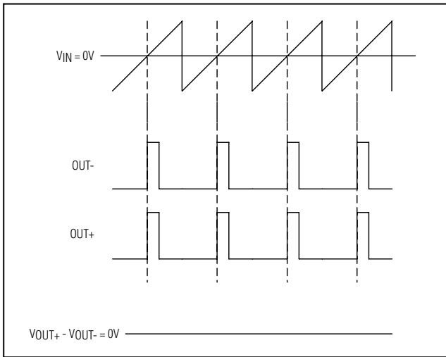
图4. 无输入信号时 MAX9770/MAX9772 的输出
