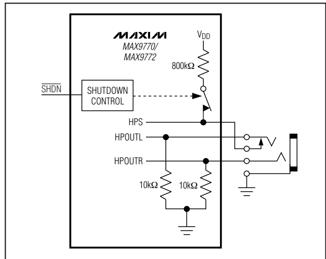
图6. HPS 配置
