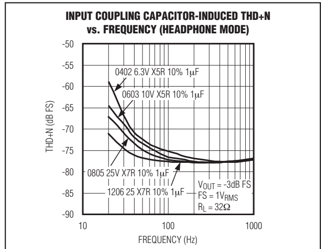
图 7. 输入耦合电容量引起的 THD+N 与频率的关系(耳机模式)
