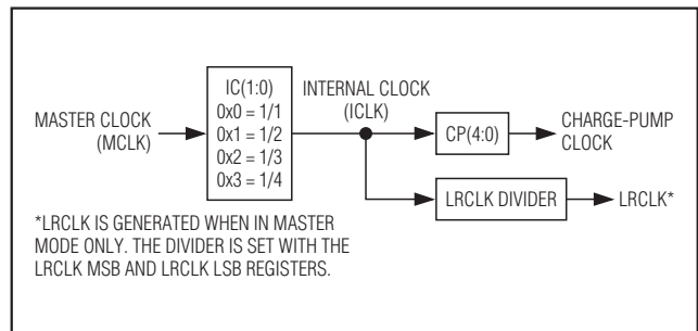
图 3. 内部时钟由 MCLK 产生
