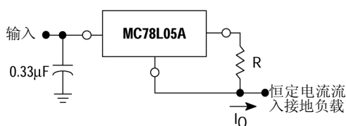
图 7. 稳流器
