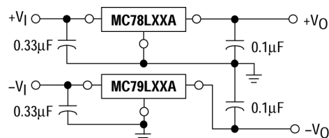
图 9. 正电压和负电压稳压器。
