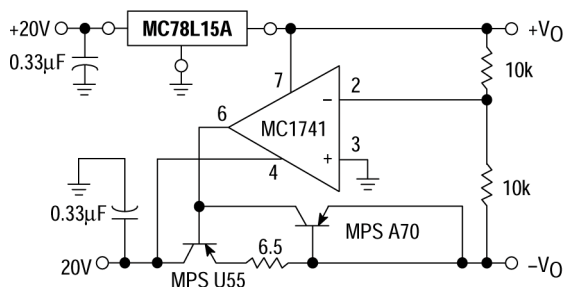
图 9. 正电压和负电压稳压器。
