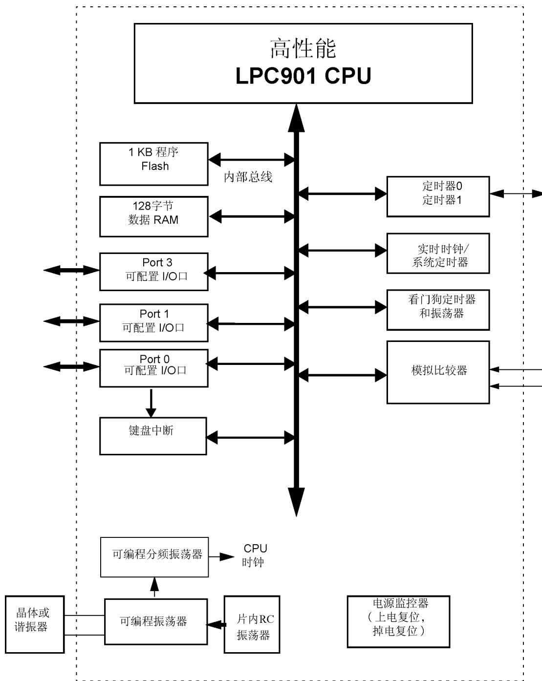
功能框图
