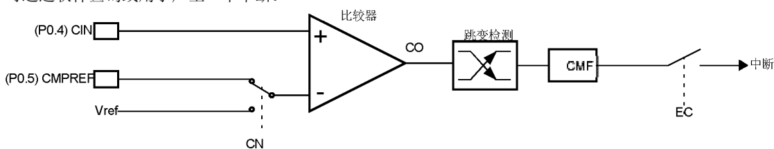
图 3 比较器输入和输出的连接
