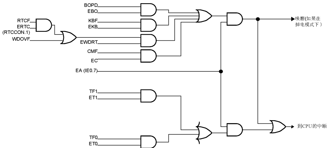
图 2 中断源, 中断使能, 掉电唤醒中断源
