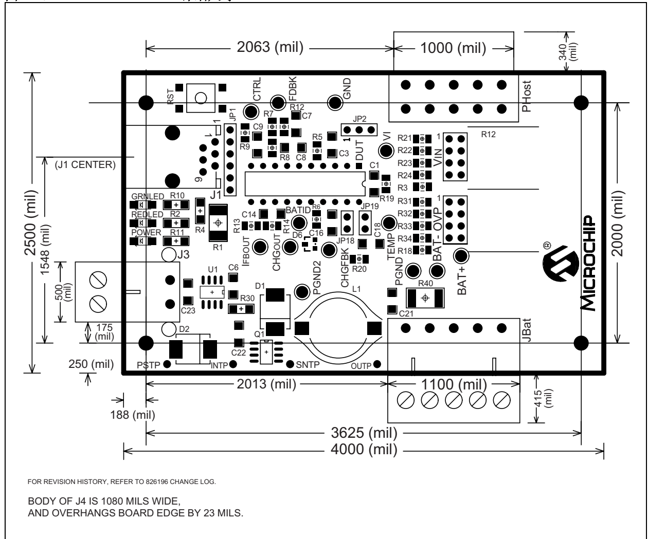
图 4-2: PS2070 详细尺寸
