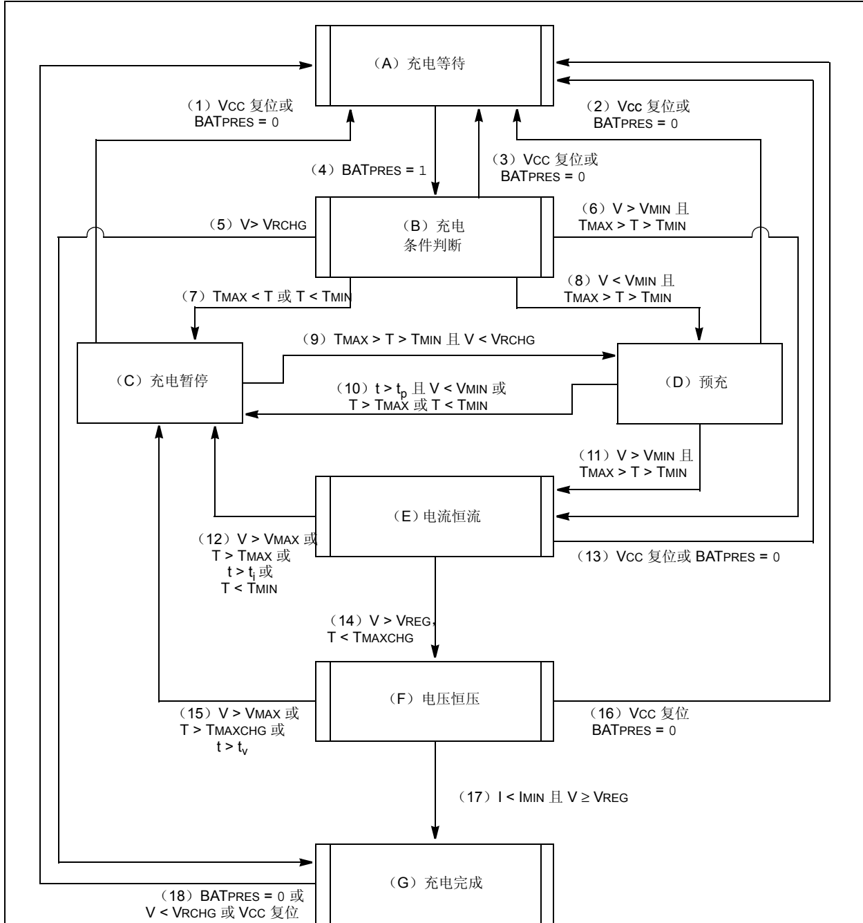
图 2-1: PS200 状态框图——锂电池充电器
