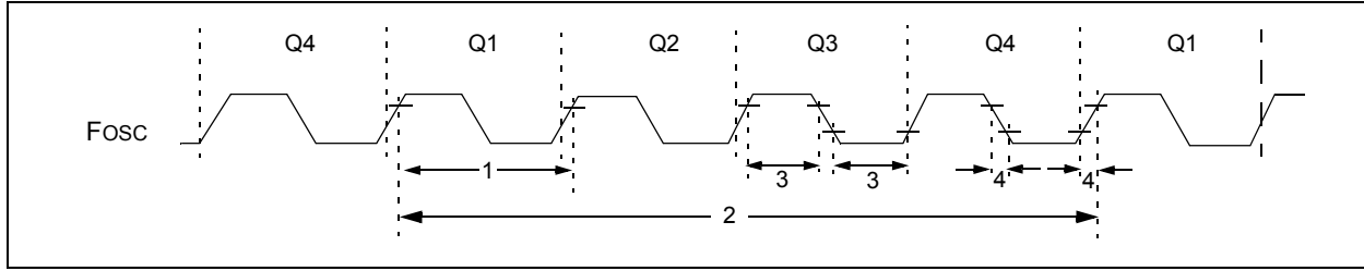
图 5-1: 外部时钟时序
