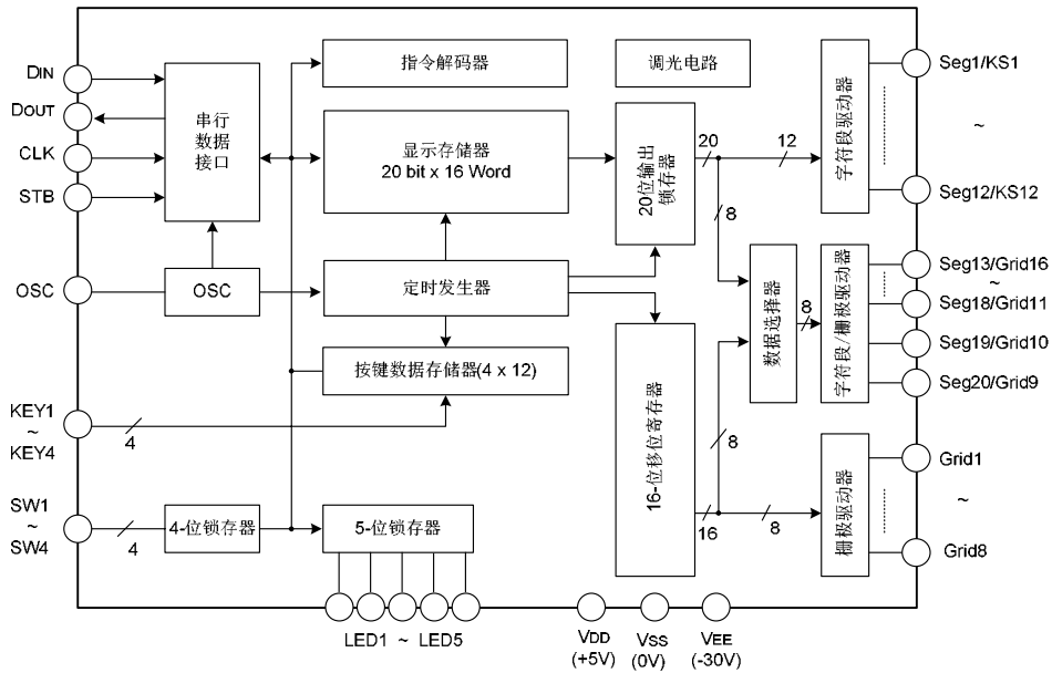
内部框图
