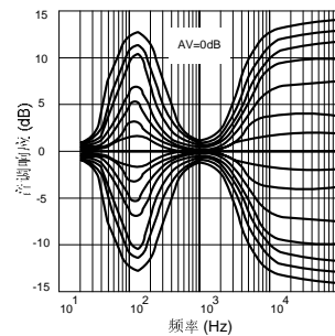
图16 典型音调响应 (用测试电路中指出的外接元件)
