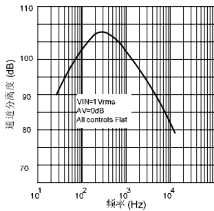
图9 通道分离度(L→R)与频率
