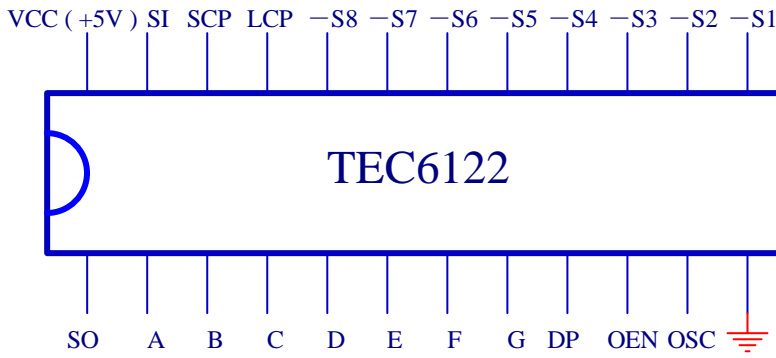
TEC6122 管脚配置图
