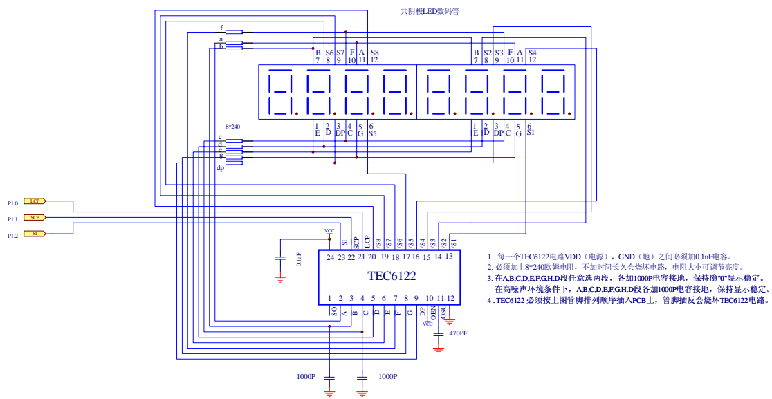
TEC6122 应用图
