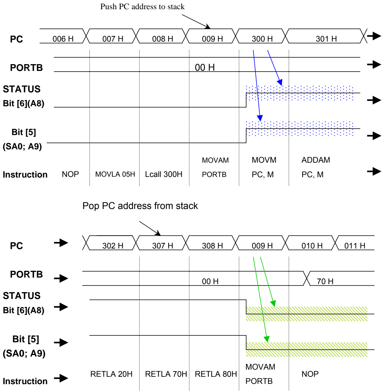
图 7-4 STATUS BIT[6:5] (页选位) 操作图
